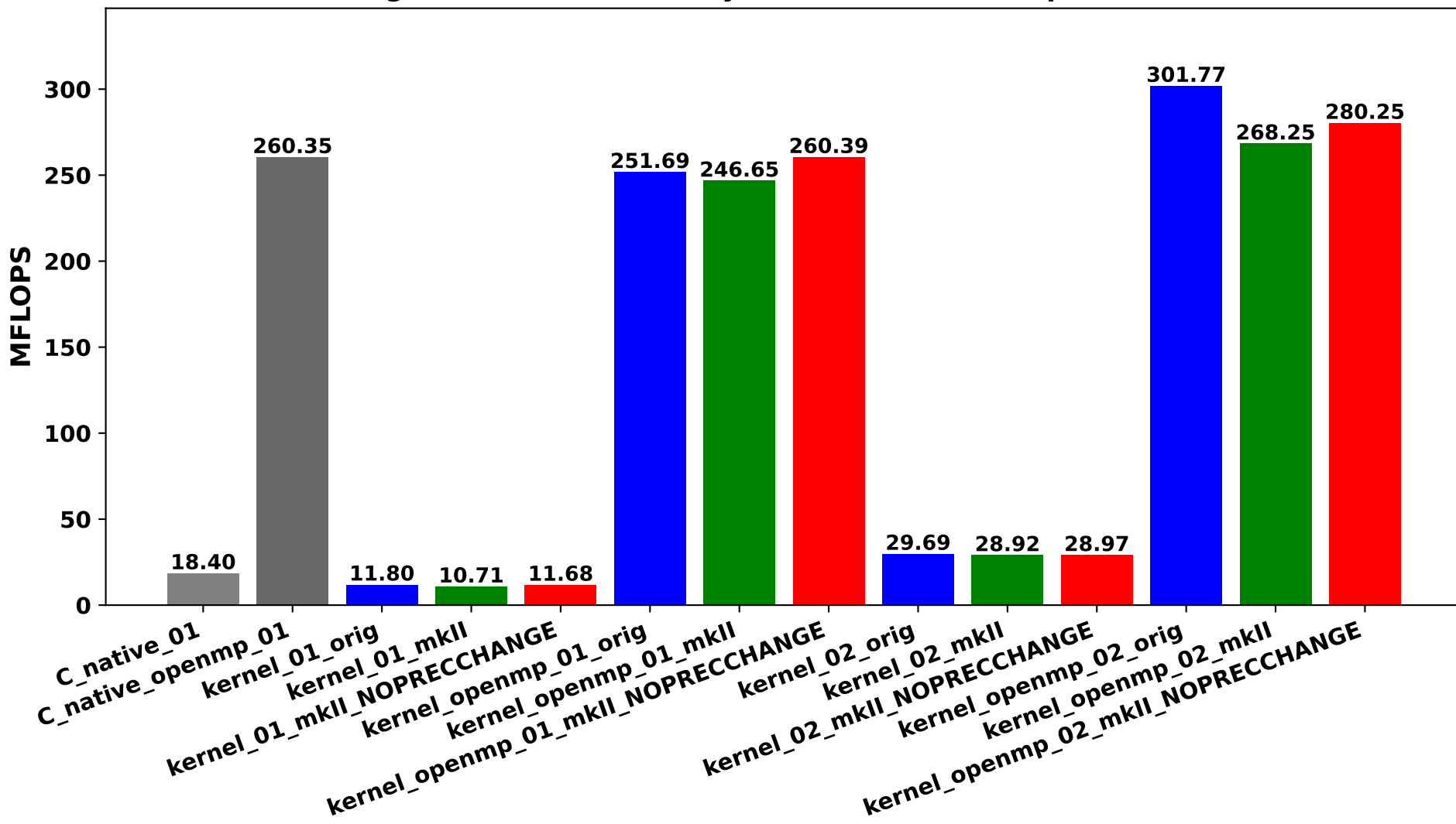
Rgemv benchmark on Ryzen 3970X 32-Core (prec=512)
