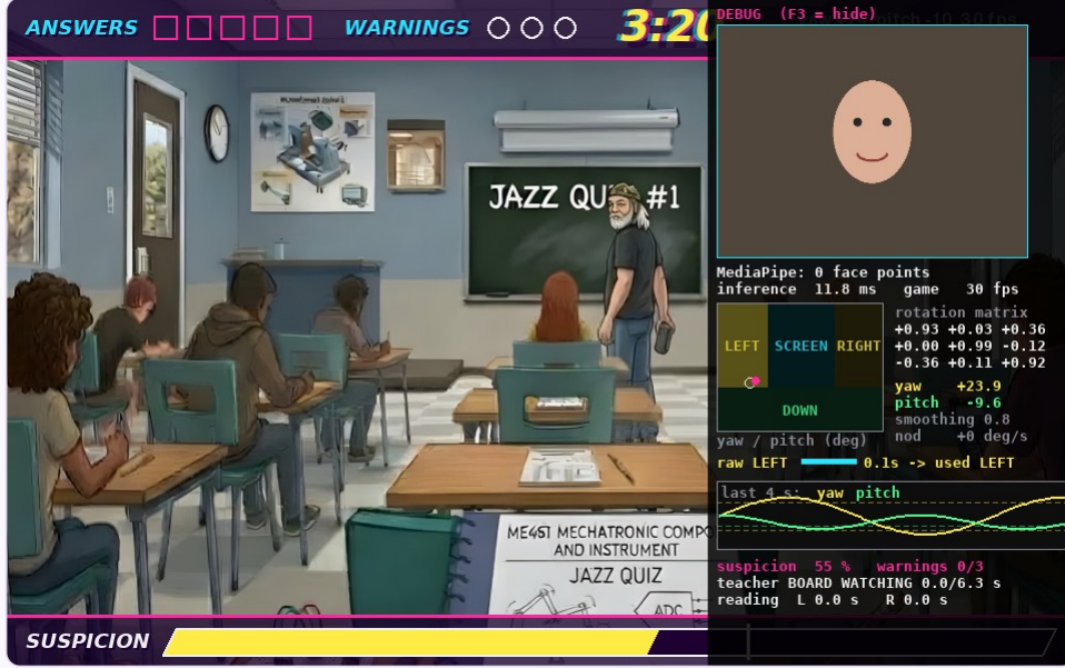
Debug paneli, oyun ekranının üstünde (örnek verilerle)
