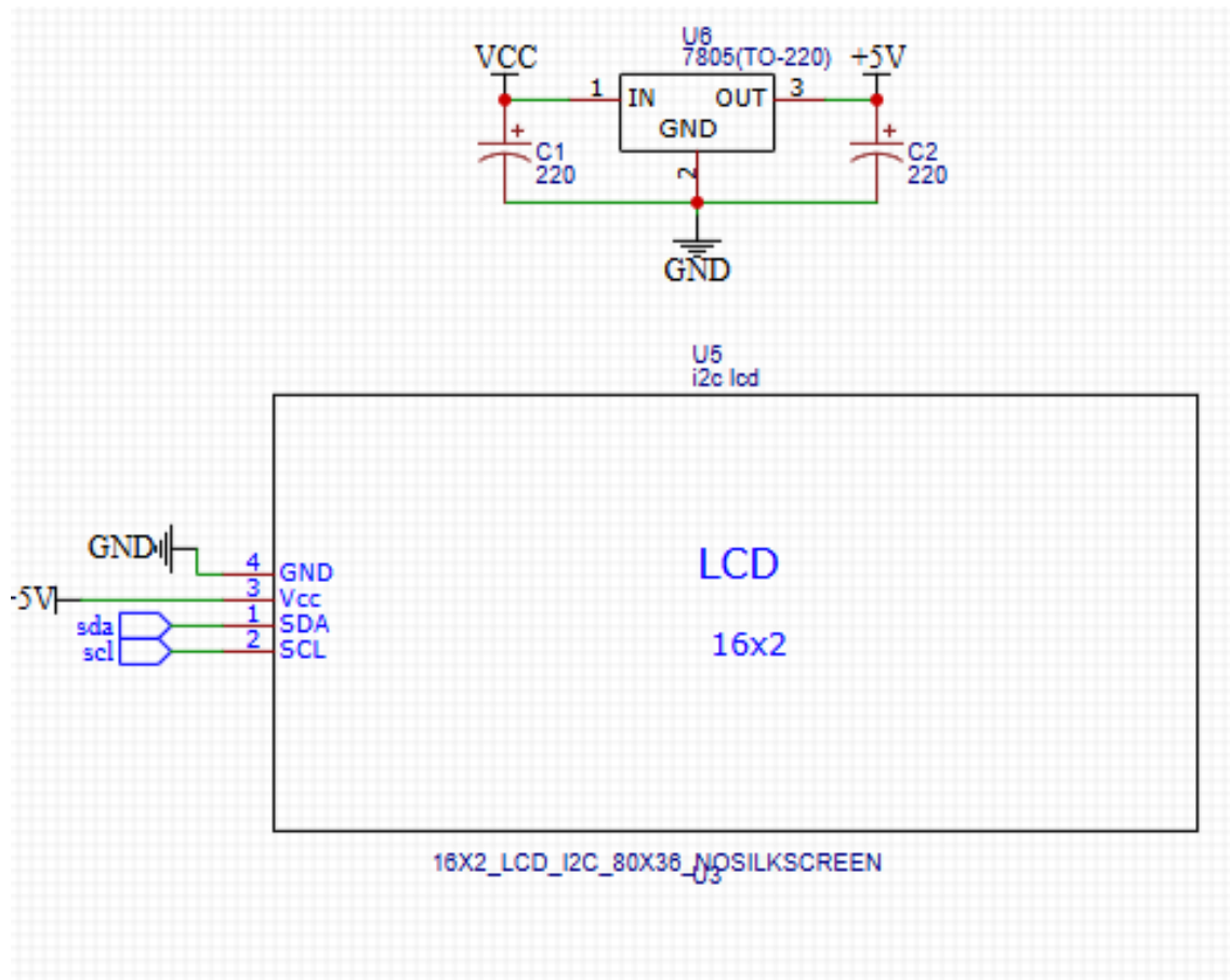
Hình 6. Nhánh 5 V ổn áp 7805 và màn hình LCD I 2 C 1602
