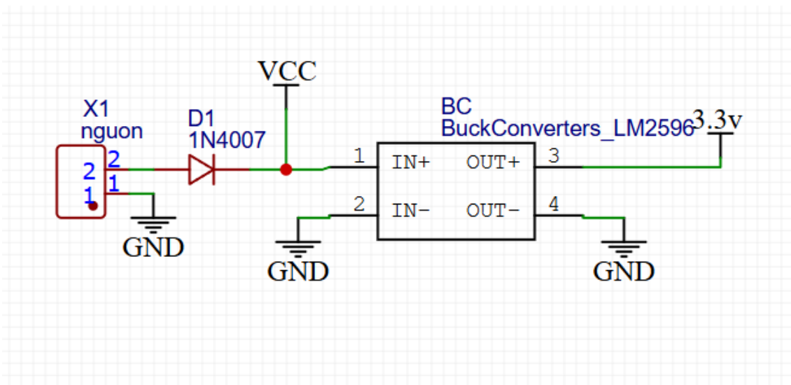
Hình 5. Mạch nguồn chống ngược cực và hạ áp LM2596
