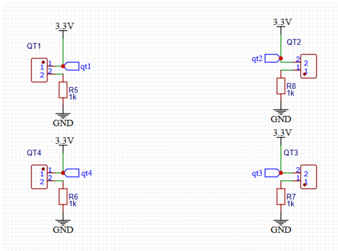
Hình 8. Mạch đọc quang trở
