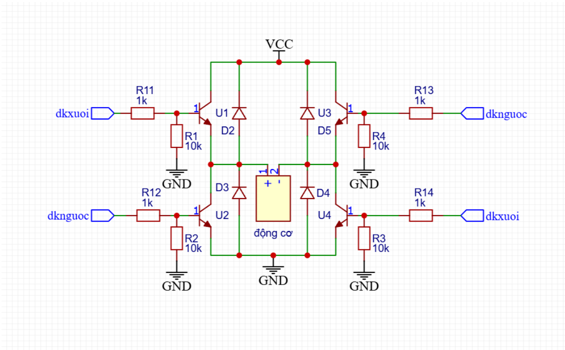
Hình 3. Mạch động lực cầu H ghép từ bốn TIP41C kèm diode bảo vệ
