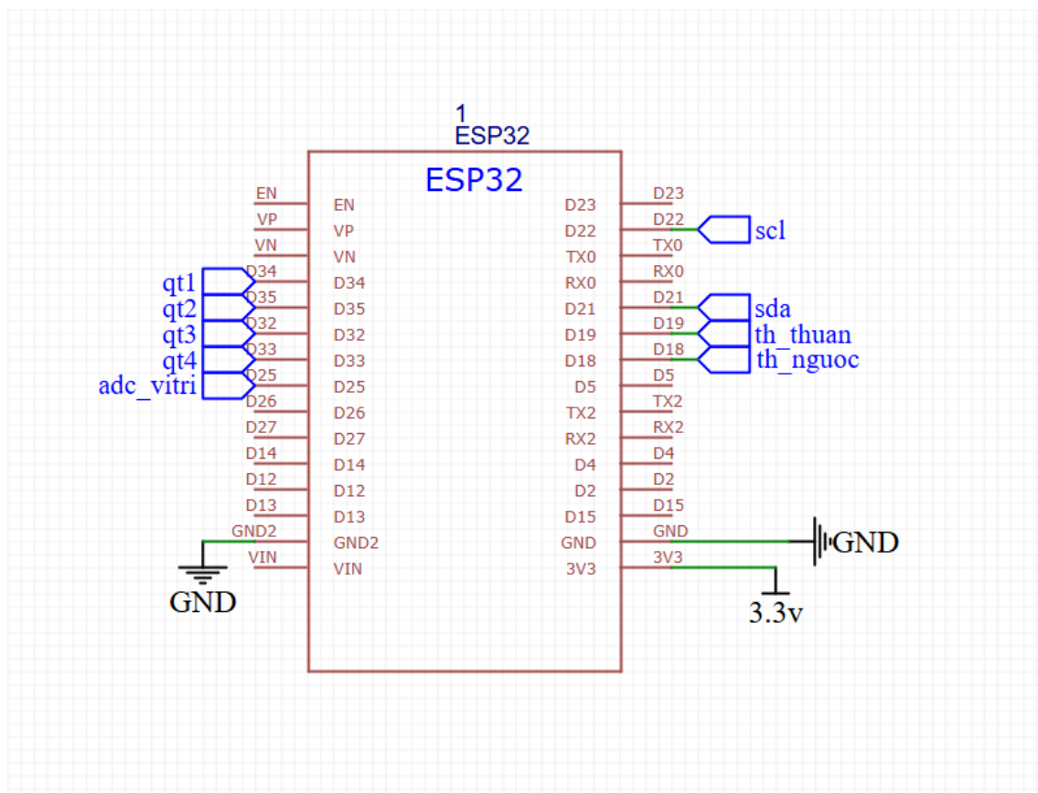
Hình 2. Sheet nguyên lý khối ESP32 DevKit và các mạng tín hiệu
