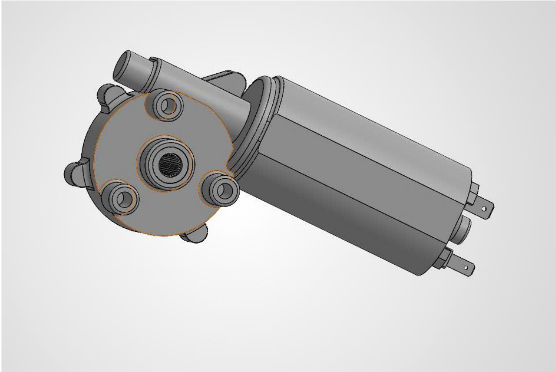
Hình 5. Động cơ gạt nước 12 V cho trục phương vị
