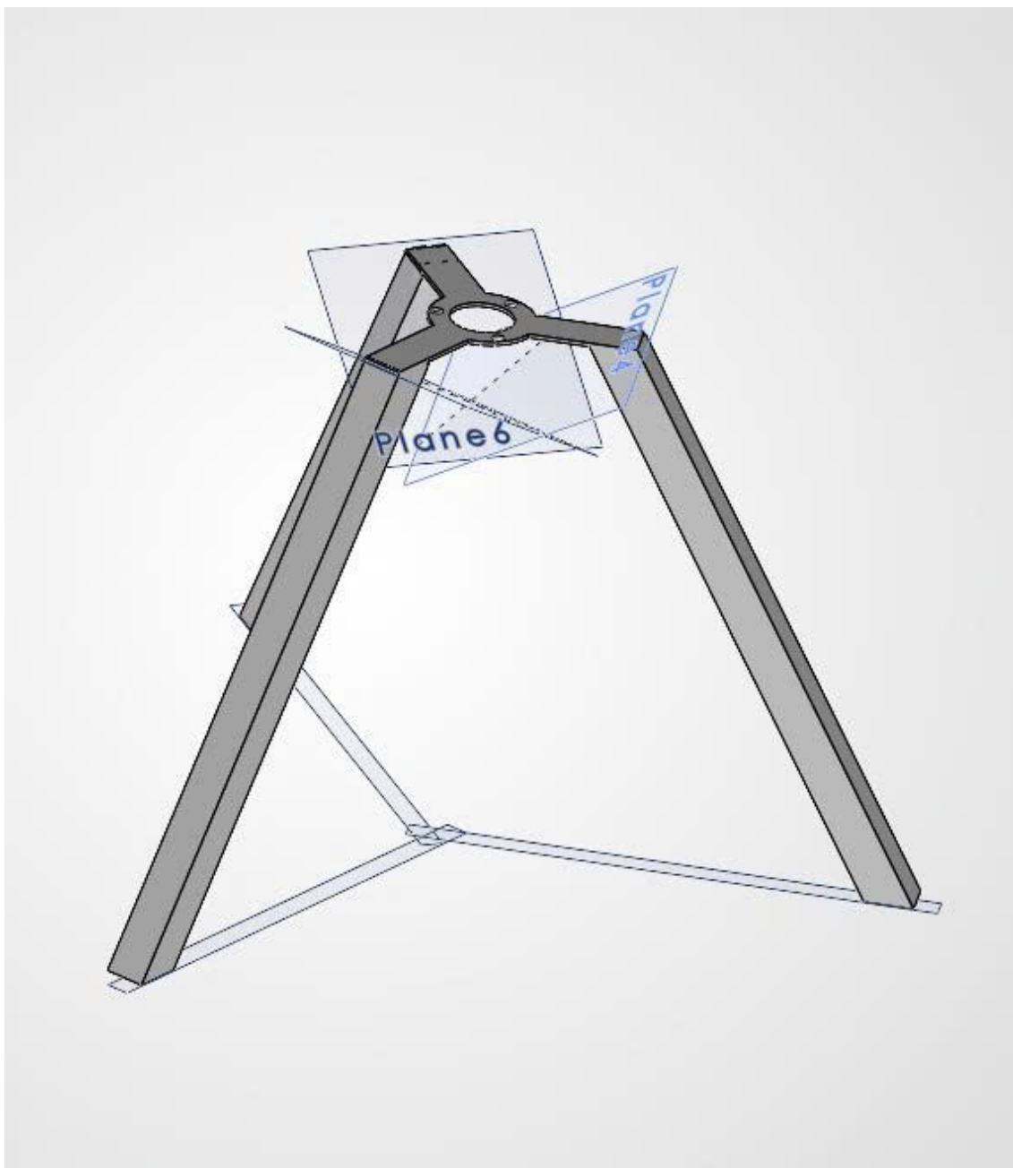
Hình 4. Chân đế ba chân và ổ khớp phương vị
