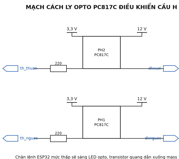
Hình 5. Cách ly opto PC817 cho từng kênh lệnh
