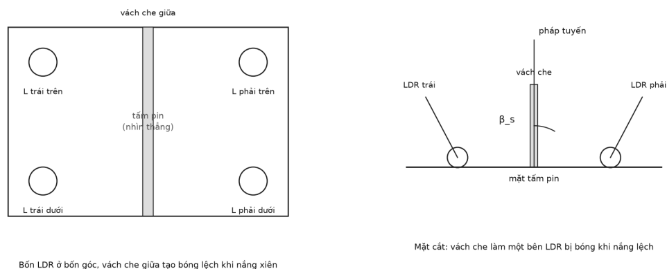
Hình 2. Bố trí bốn LDR và vách che giữa trên tấm pin
