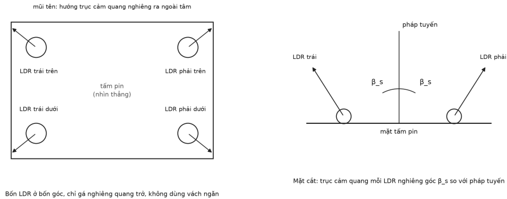
Hình 2. Bốn LDR gá nghiêng \beta_s ở bốn góc tấm pin, không dùng vách ngăn
