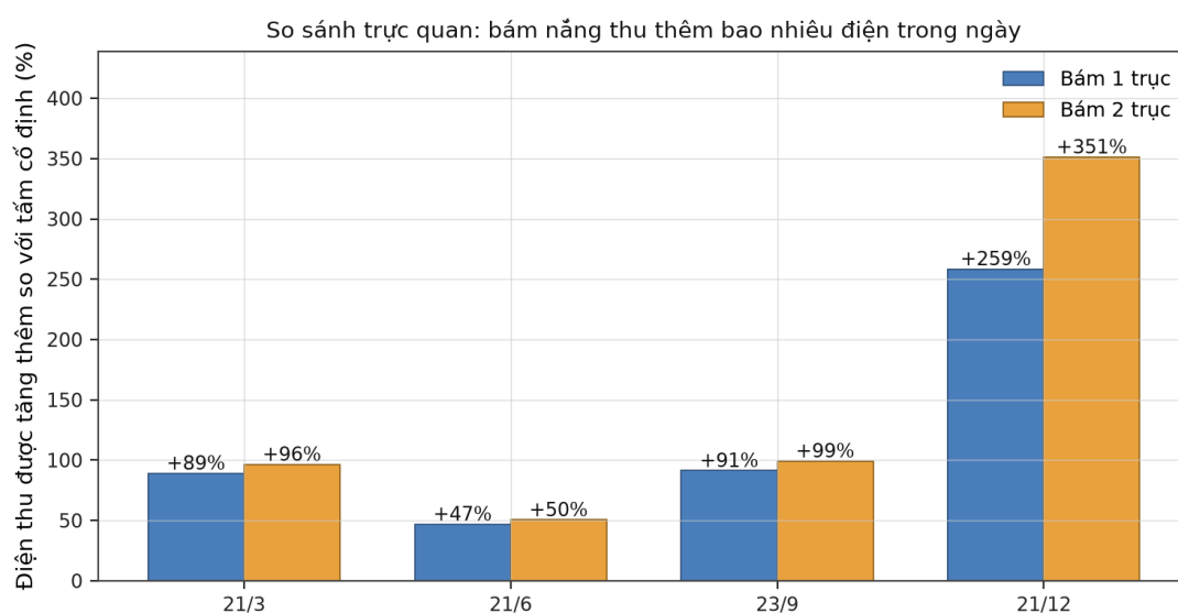
Hình 4. Phần trăm điện thu thêm so với tấm cố định trong bốn ngày đại diện (mô phỏng tham khảo, sẽ kiểm chứng)
