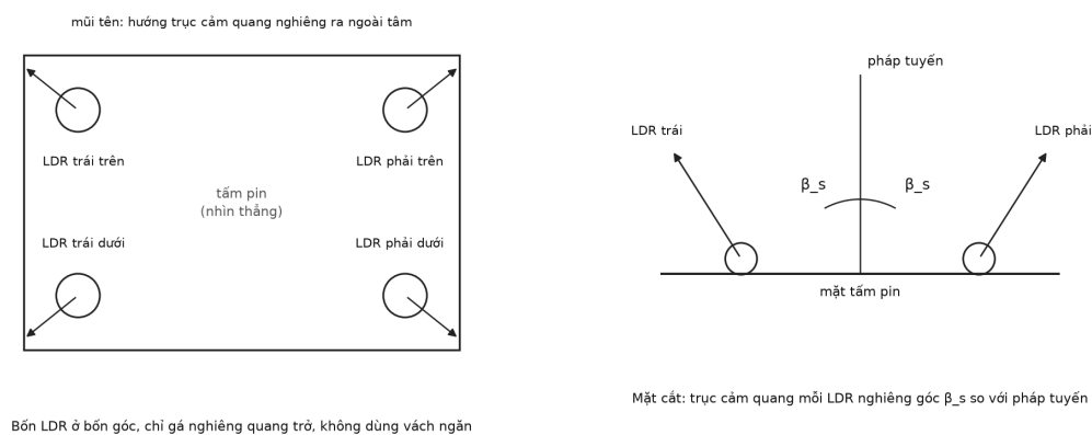
Hình 2. Bố trí bốn LDR gá nghiêng \beta_s trên tấm pin hai trục
