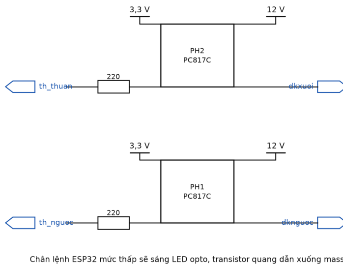
MẠCH CÁCH LY OPTO PC817C ĐIỀU KHIỂN CẦU H
