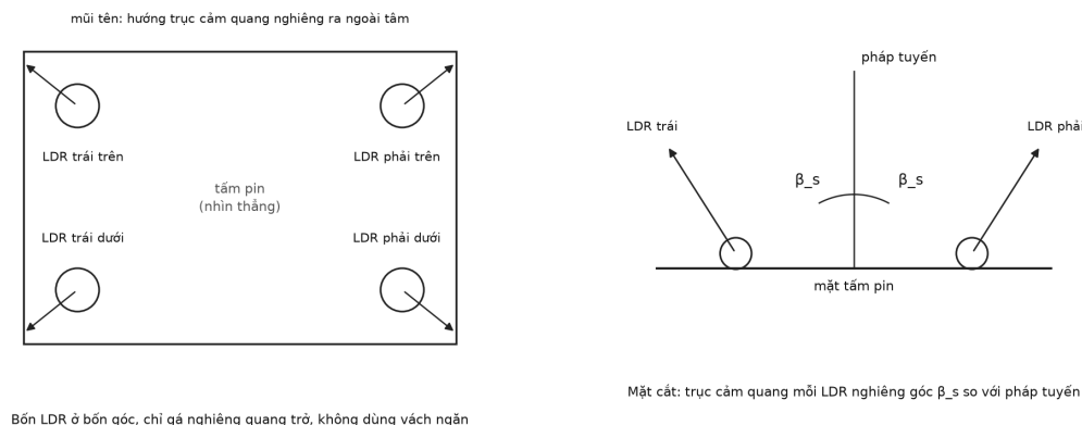
Hình 2. Bố trí bốn LDR gá nghiêng \beta_s trên tấm pin
