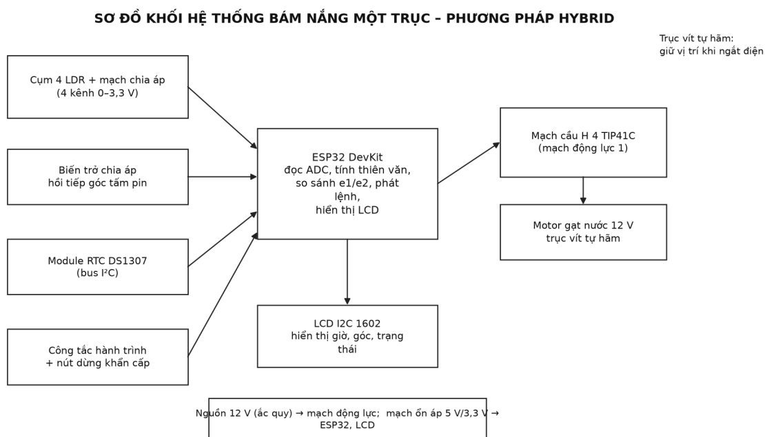
Hình 1. Sơ đồ khối hệ thống bám năng một trục phương pháp hybrid
