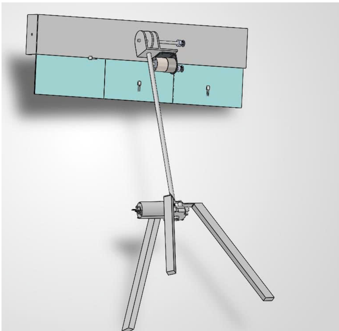
Hình 3. Toàn cảnh cơ cấu bám hai trục nhìn từ phía sau
