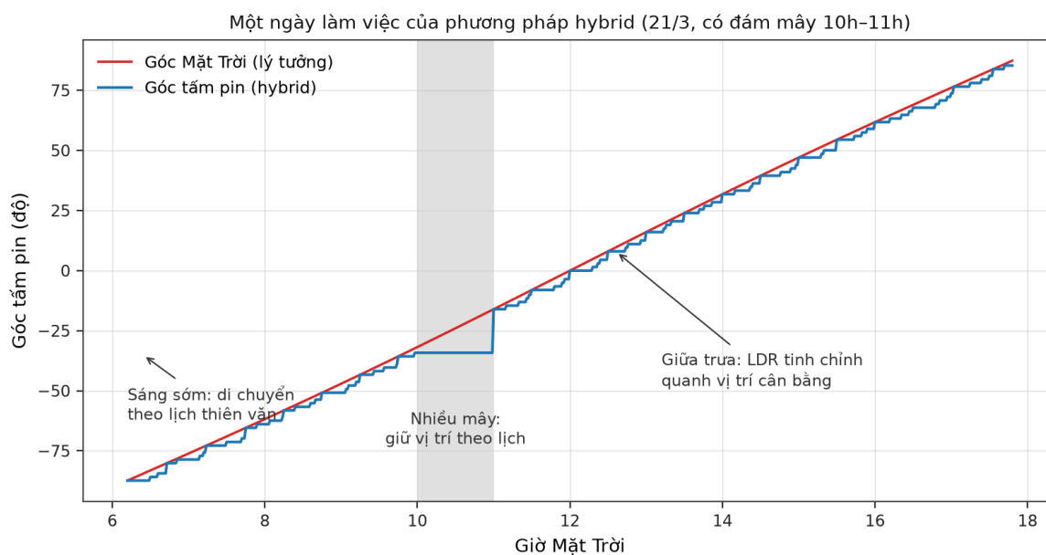
Hình 3. Góc tấm pin theo thời gian ngày 21/3 của luật hybrid (trực phương vị)
