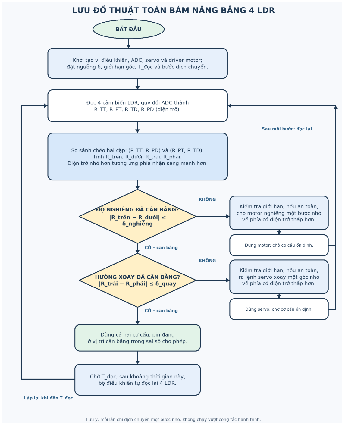
Hình 5. Lưu đồ thuật toán bám nắng bằng bốn LDR do sinh viên vẽ
