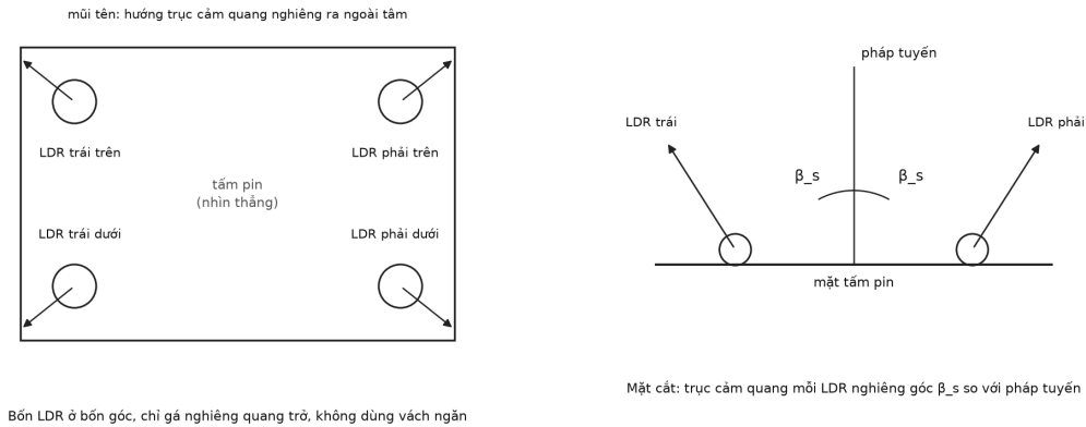
Hình 2. Bốn LDR gá nghiêng \beta_s ở bốn góc tấm pin hai trục
