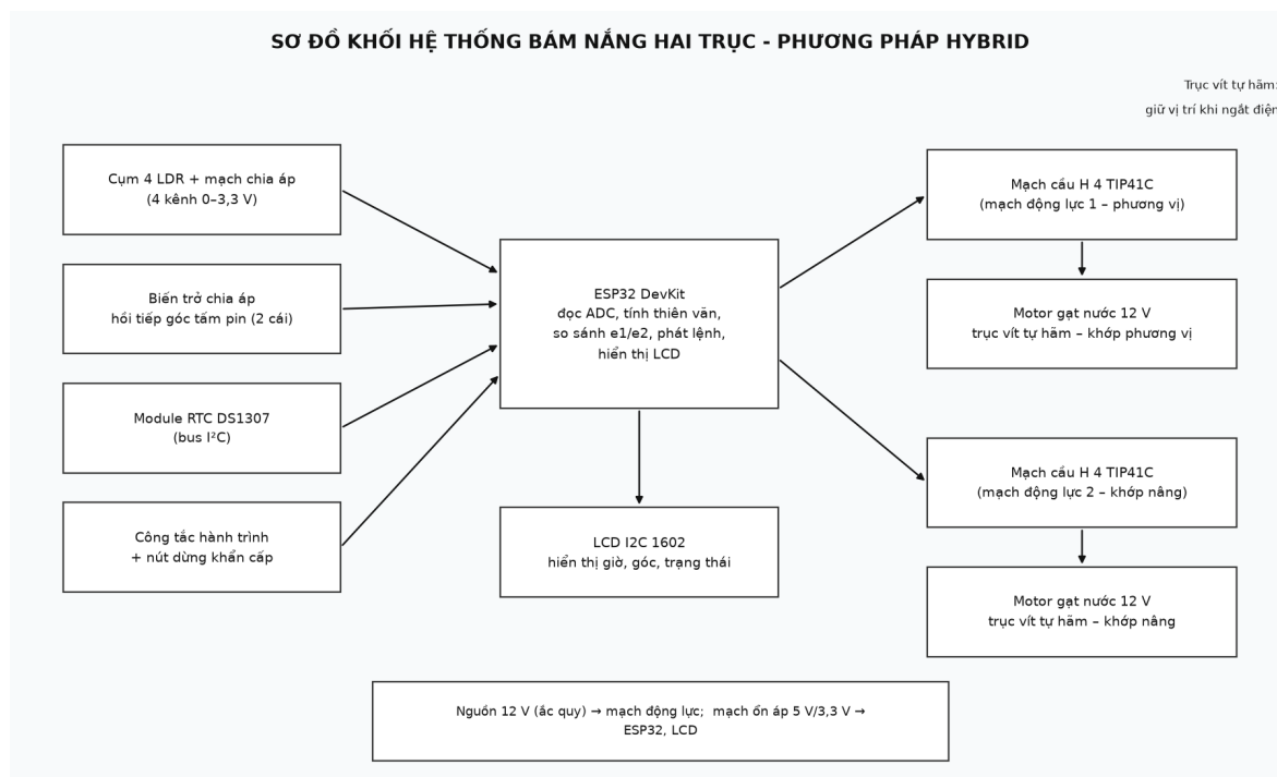
Hình 1. Sơ đồ khối hệ thống hai trục theo phương pháp hybrid
