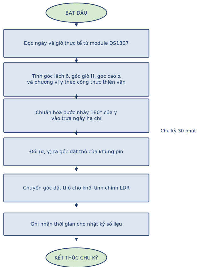
Hình 2. Lưu đồ đọc giờ DS1307 và tính góc thiên văn
