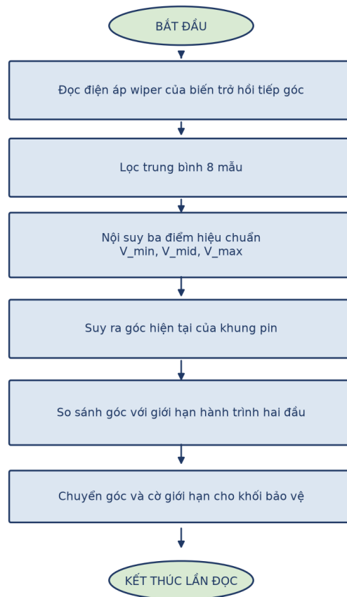
Hình 6. Lưu đồ đọc biến trở suy ra góc khớp
