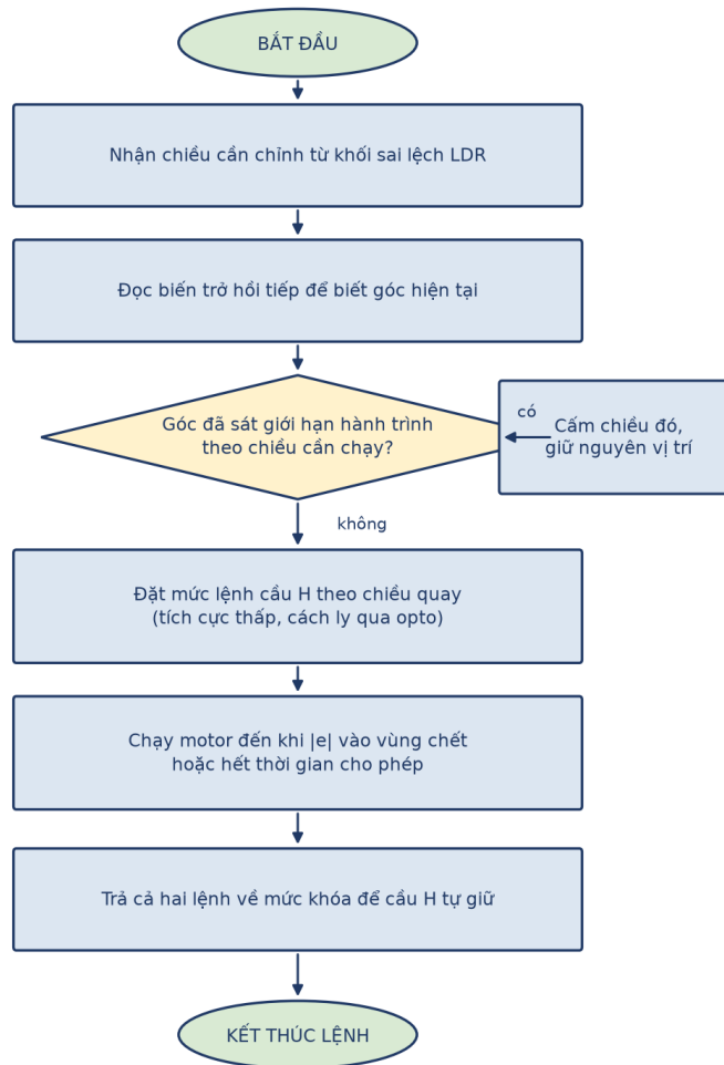
Hình 4. Lưu đồ điều khiển motor qua cầu H bốn TIP41C
