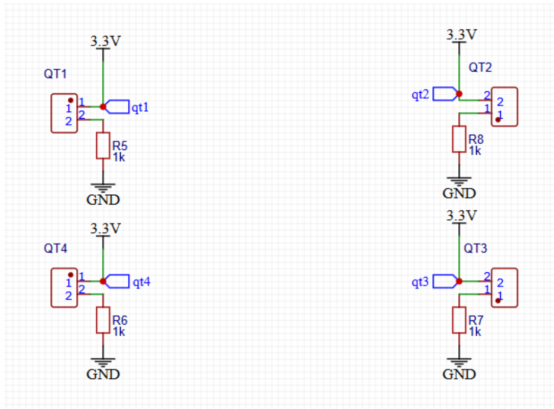
Hình 8. Mạch đọc quang trở
