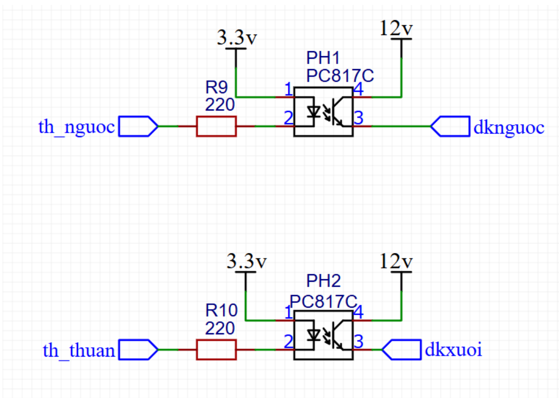
Hình 4. Mạch cách ly opto PC817 giữa khối điều khiển và mạch động lực
