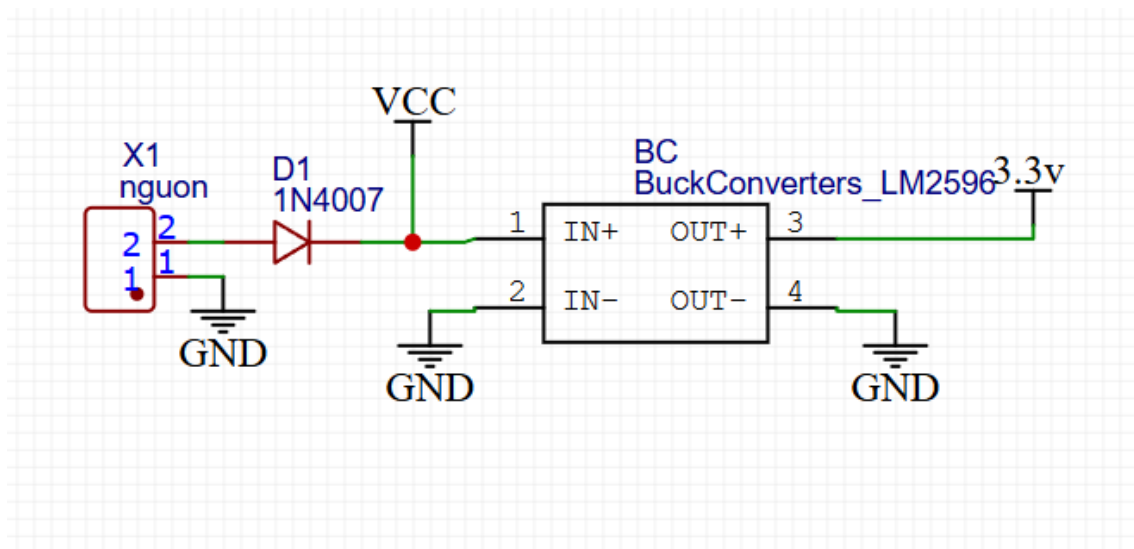
Hình 5. Mạch nguồn chống ngược cực và hạ áp LM2596
