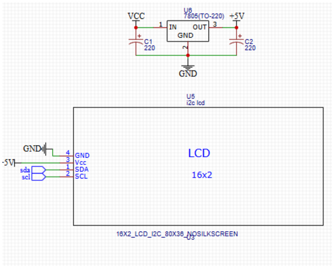
Hình 6. Nhánh 5 V ổn áp 7805 và màn hình LCD I 2 C 1602
