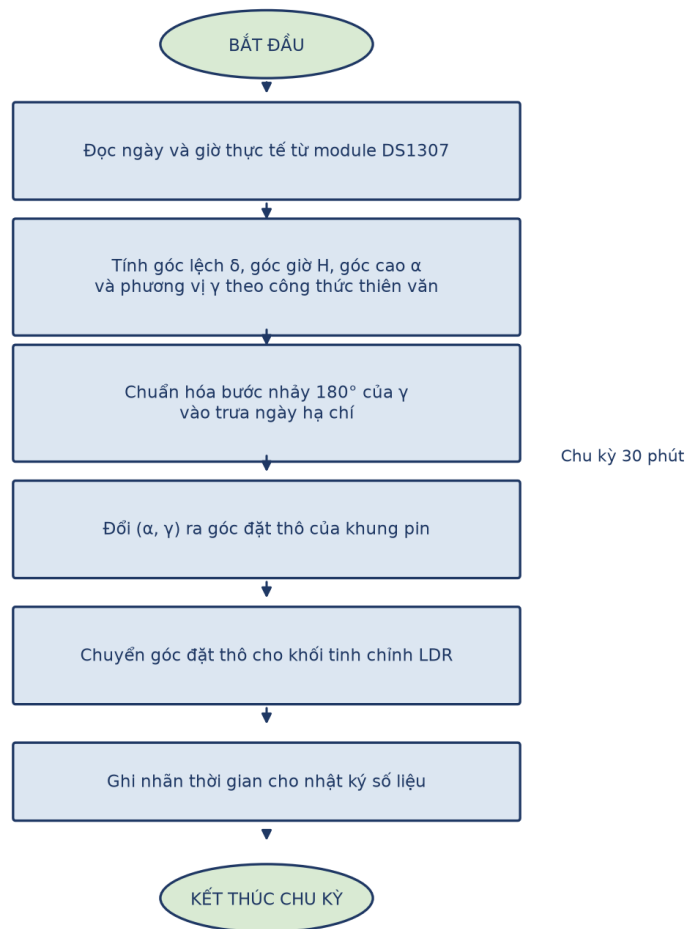
Hình 1. Lưu đồ đọc giờ DS1307 và tính góc thiên văn
