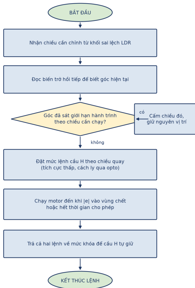
Hình 3. Lưu đồ điều khiển motor qua cầu H bốn TIP41C
