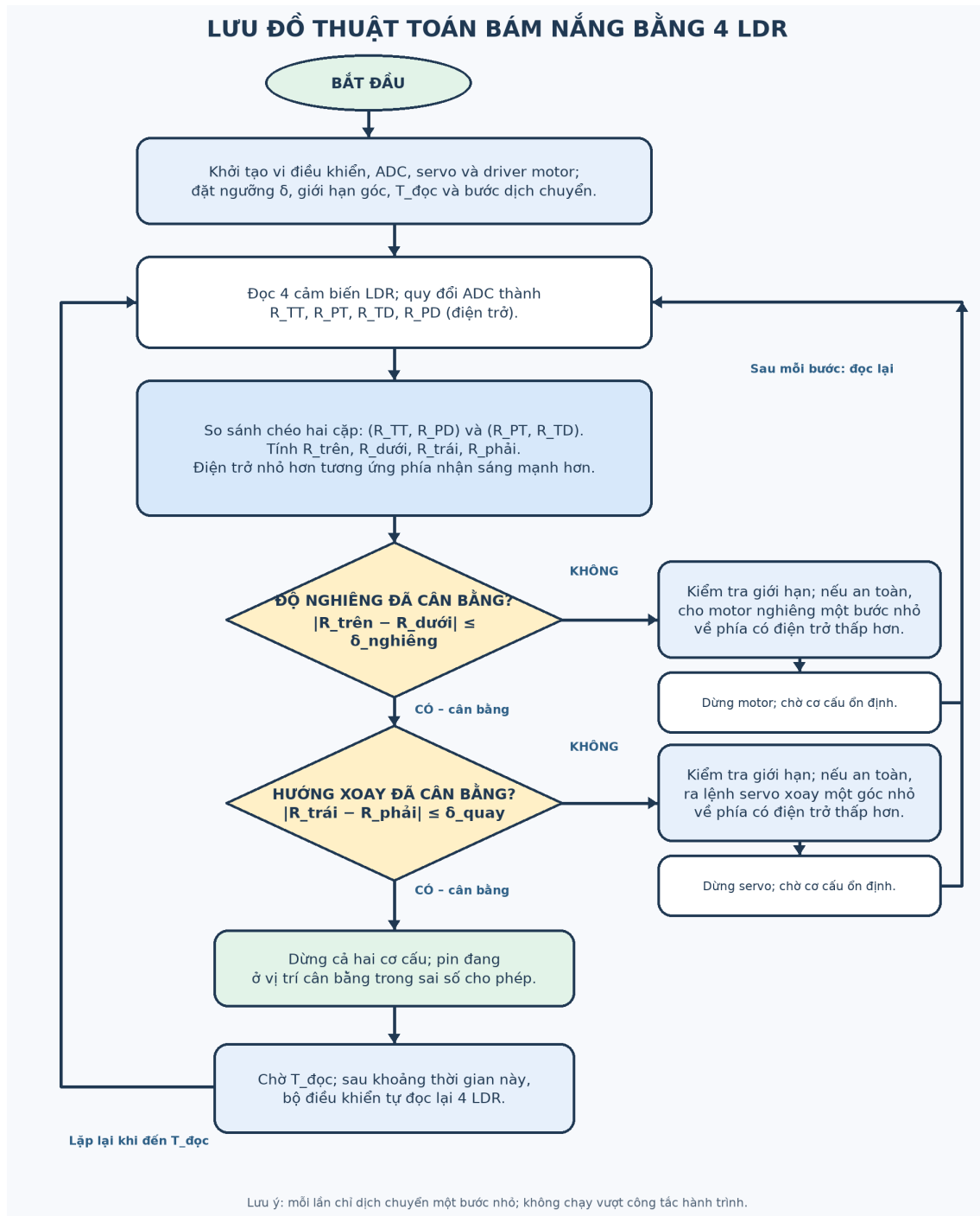
Hình 5. Lưu đồ thuật toán bám năng bằng bốn LDR do sinh viên vẽ
