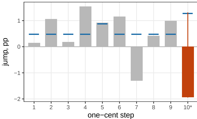
(d) roundness fit (blue) and the estimate (arrow)
