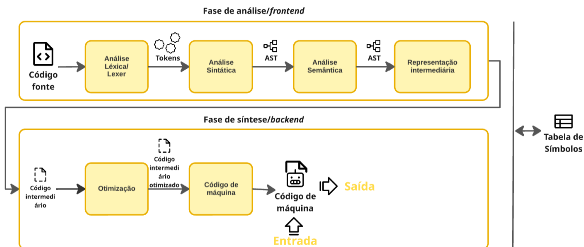
Figura 05 - Módulos e fases de um compilador
