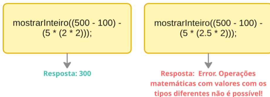
Figura 25 - Códigos-fonte do NiloScript corretos e incorretos
