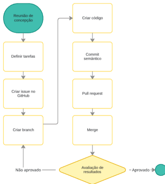
Figura 21 - Exemplo de diagrama de fluxo de trabalho do NiloScript
