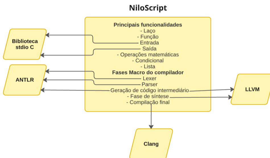
Figura 09 - Estruturas e ferramentas do NiloScript.
