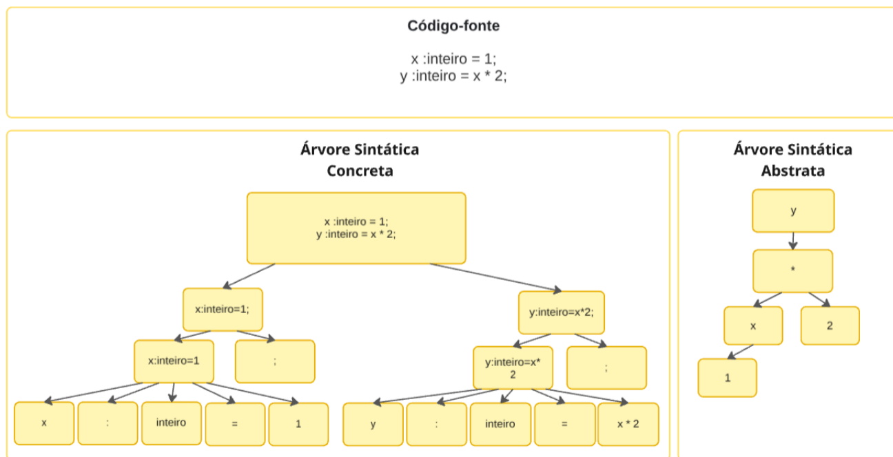
Figura 10 - Comparação de uma árvore sintática abstrata e uma concreta de um código-fonte NiloScript.
