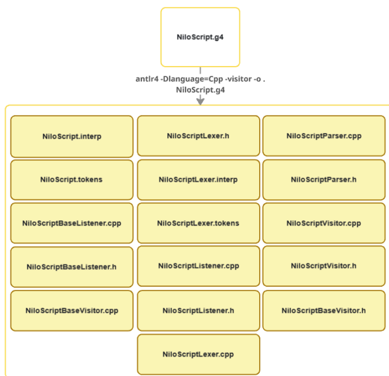
Figura 27 - Comando utilizado para gerar lexer e parser a partir da gramática.
