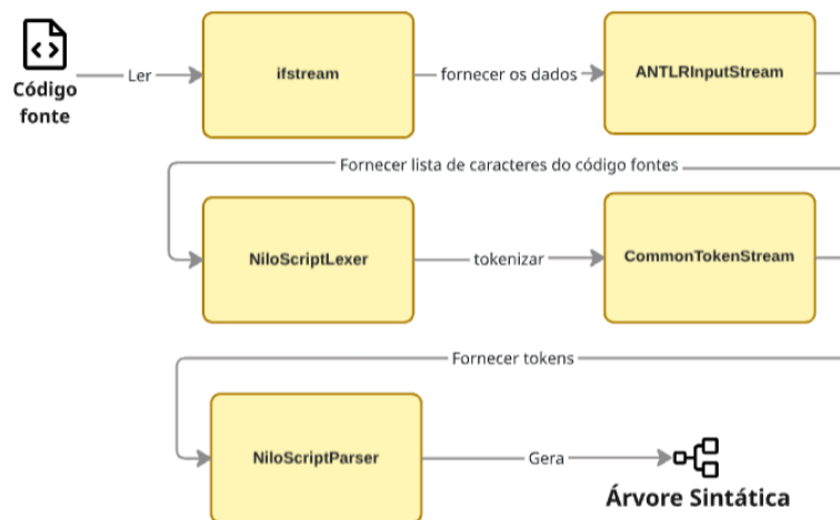
Figura 28 - Comandos utilizados para a geração de uma árvore sintática a partir de um código-fonte.
