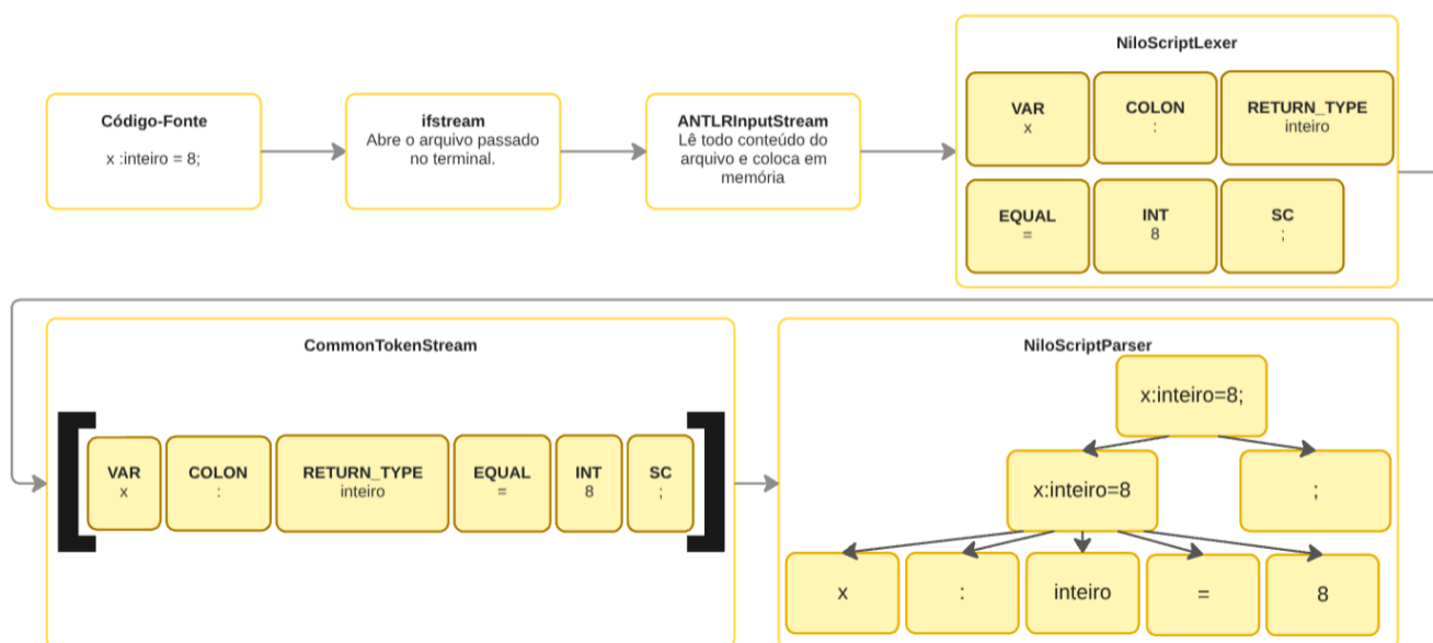
Figura 29 - Exemplo do fluxo completo de comandos partindo de um código-fonte
