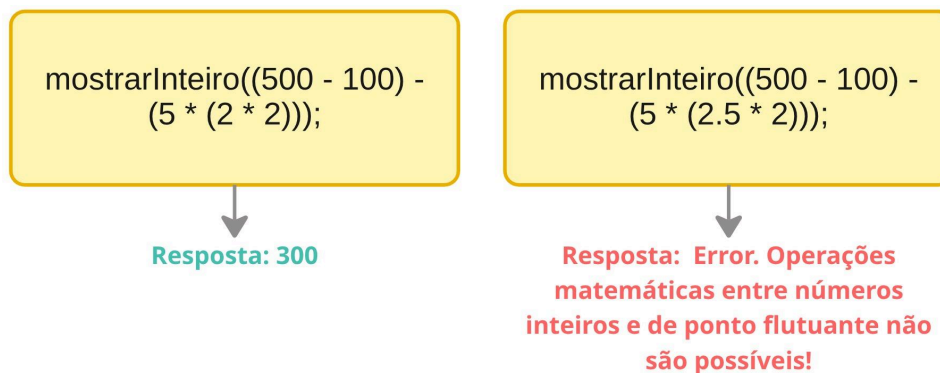
Figura 33 - Códigos-fonte do NiloScript corretos e incorretos
