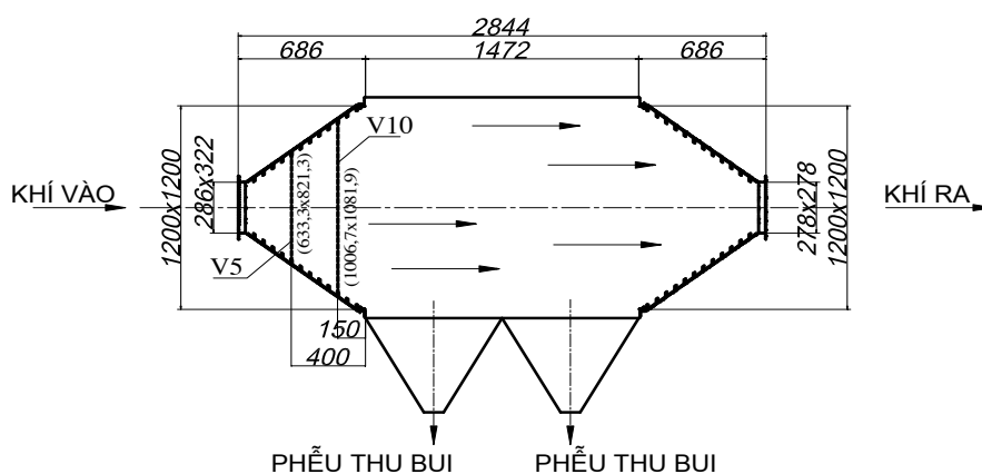
Hình 4.7a. Sơ đồ V10:V5 \Rightarrow đầu ra không lười
