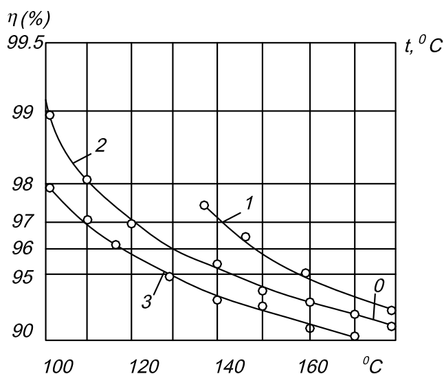
Hình 1.14. Đồ thị sự ảnh hưởng của nhiệt độ tới hiệu suất lọc bụi[39]
