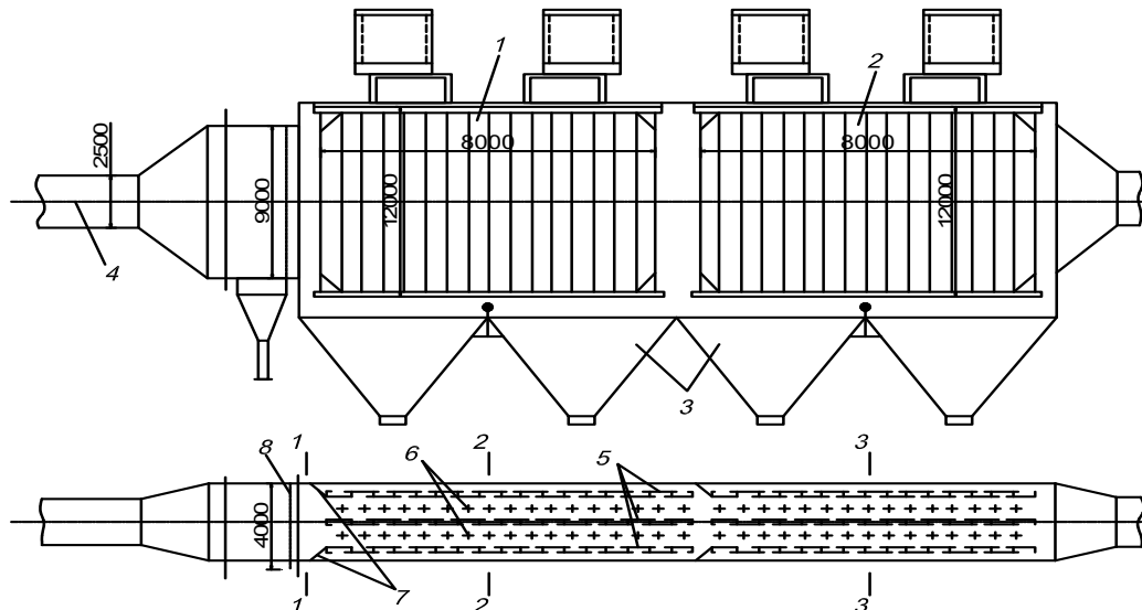
Hình 4.19. Mô hình thiết bị lọc bụi tĩnh điện công nghiệp Q/2DC-31
