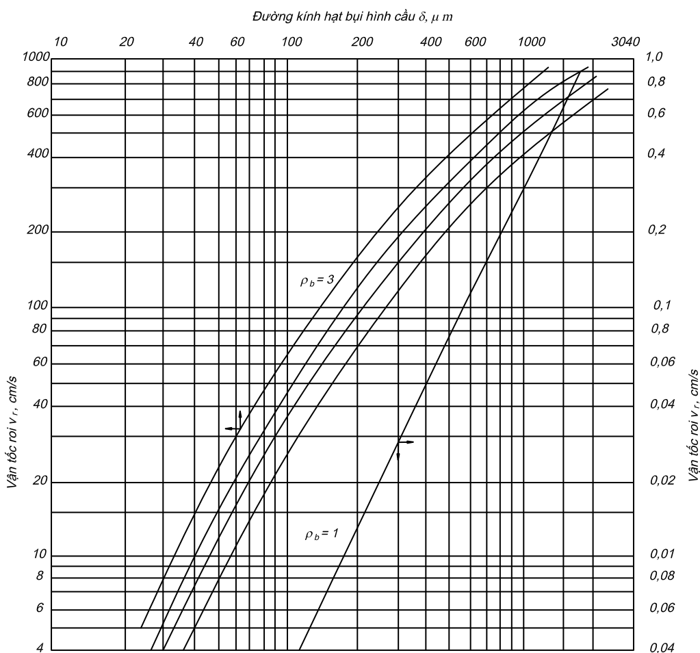
Hình 2.3. Biểu đồ vận tốc rơi: Giới hạn của hạt thực tế trong không khí ở nhiệt độ 20^\circ C tương ứng với khối lượng đơn vị của bụi \rho = 1-3 g/cm^3 [3].
