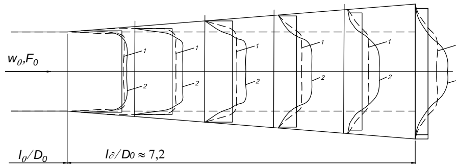
Hình 2.9. Biểu đồ trường vận tốc trên các tiết diện khác nhau của đoạn kênh mở rộng, \alpha_1 = 8^\circ , F_1/F_0 = 4 , [14, 15]
