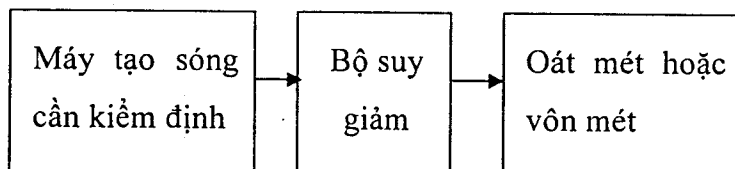
Hình 2 : Sơ đồ kiểm tra mức ra cực đại
