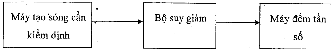
Hình 1: Sơ đồ kiểm tra sai số thiết lập tần số, kiểm tra độ không ổn định tần số tín hiệu
