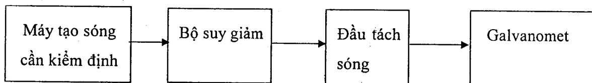
Hình 3: Sơ đồ kiểm tra giới hạn điều chỉnh mức tín hiệu
