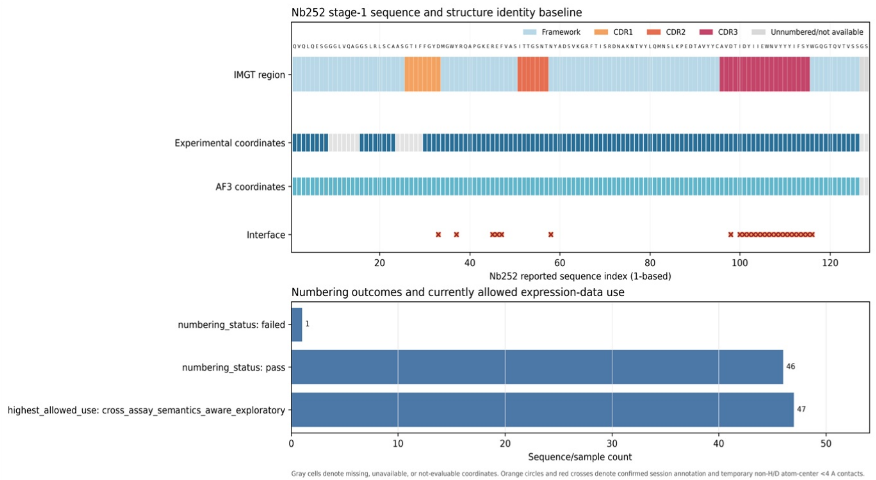
图 2 序列、实验坐标覆盖、AF3 坐标覆盖及实验界面位置基线。灰色代表实验坐标不可评价，不等同于序列缺失。
