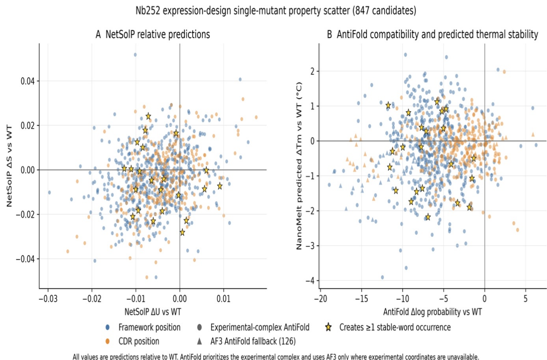
图9 四指标关键组合散点图。点形区分 AntiFold 实验复合物视图与 AF3 单体补充视图；星号标记稳定词新增。
