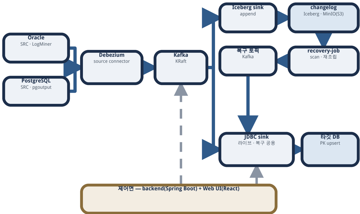
그림 A. 전체 아키텍처 — 캡처(소스별) → Kafka → 실적재(JDBC sink)·changelog(Iceberg sink) 병행, 복구는 changelog → recovery-job → 복구 토픽 → 동일 JDBC sink로 합류. 점선은 제어면의 배포·관리 경로.
