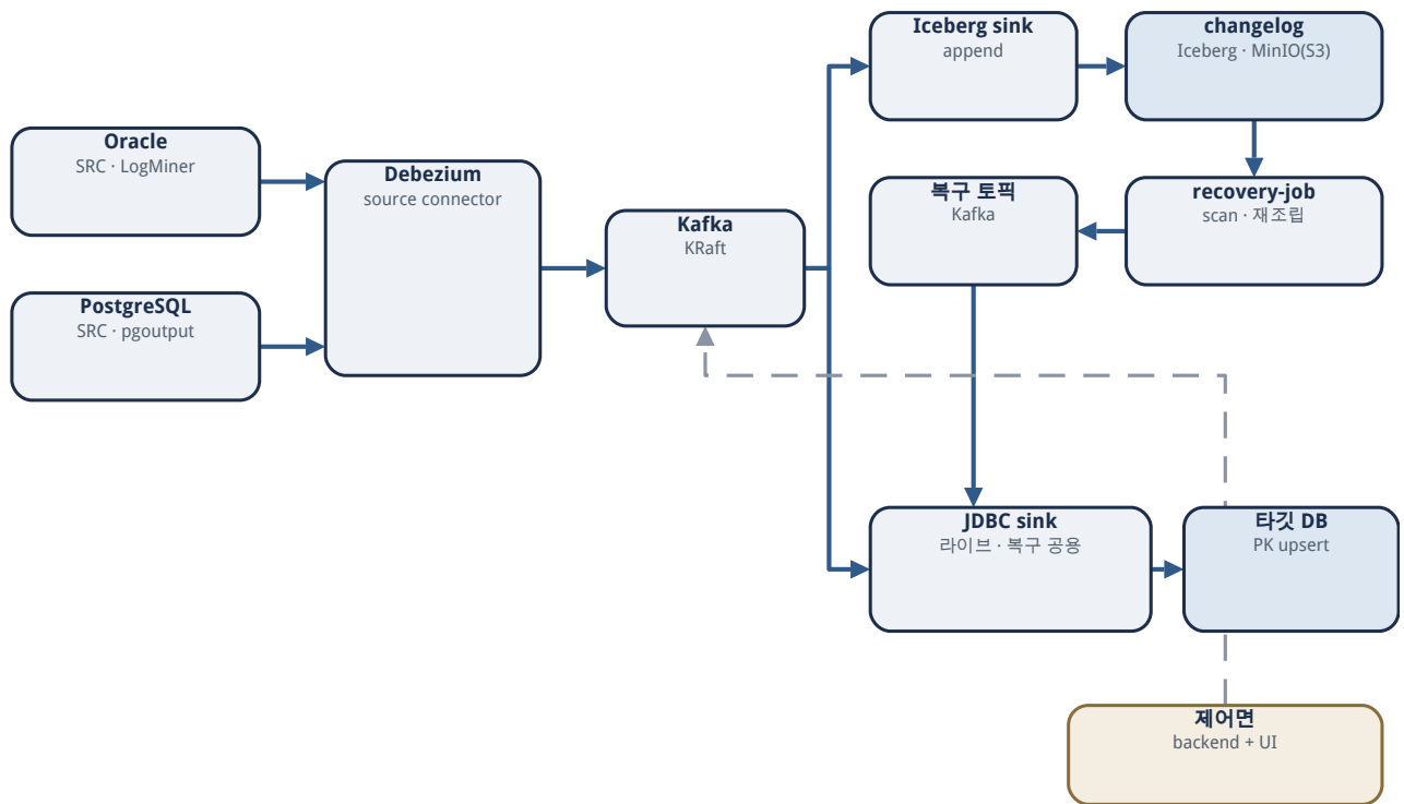
그림 A. 전체 아키텍처 — 캡처(소스별) → Kafka → 실적재(JDBC sink)·changelog(Iceberg sink) 병행, 복구는 changelog → recovery-job → 복구 토픽 → 동일 JDBC sink로 합류. 점선은 제어면의 배포·관리 경로.
