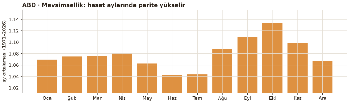
Şekil 4 · Ay ortalamaları, 1971-2026.
