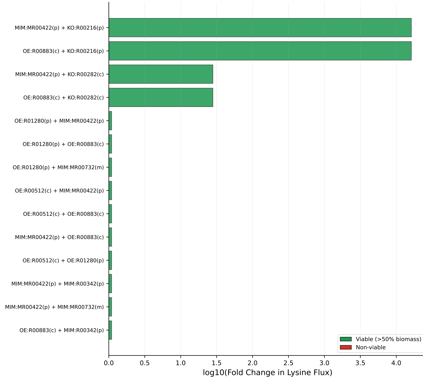
A. Top Combination Strategies
