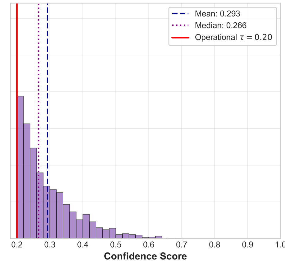
YOLO26m (N = 1,484)
