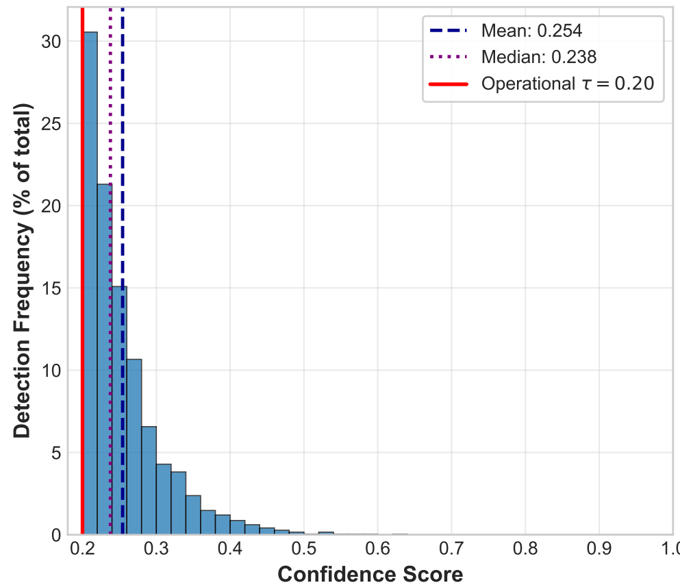
YOLO26n (N = 5,084)
