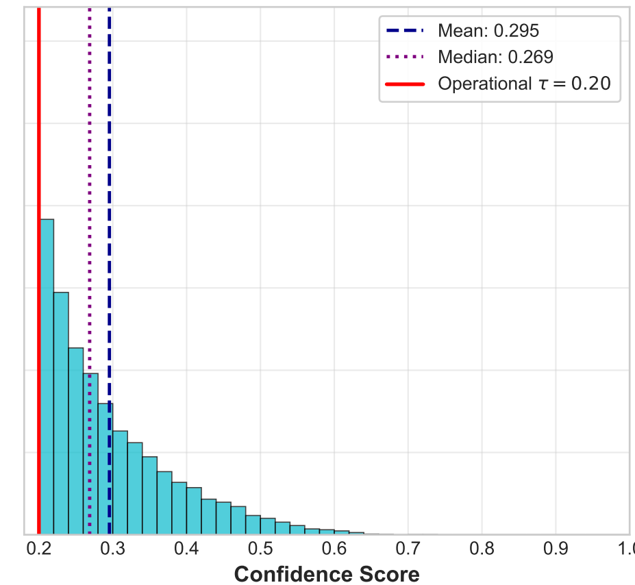
YOLO26s (N = 14,102)
