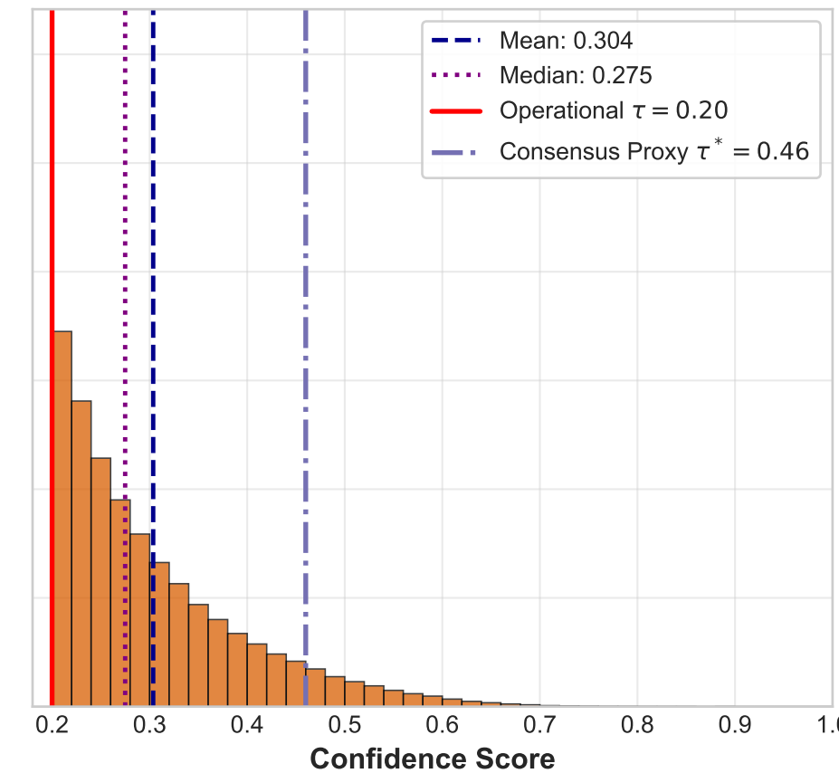
YOLOv8n (N = 353,427)
