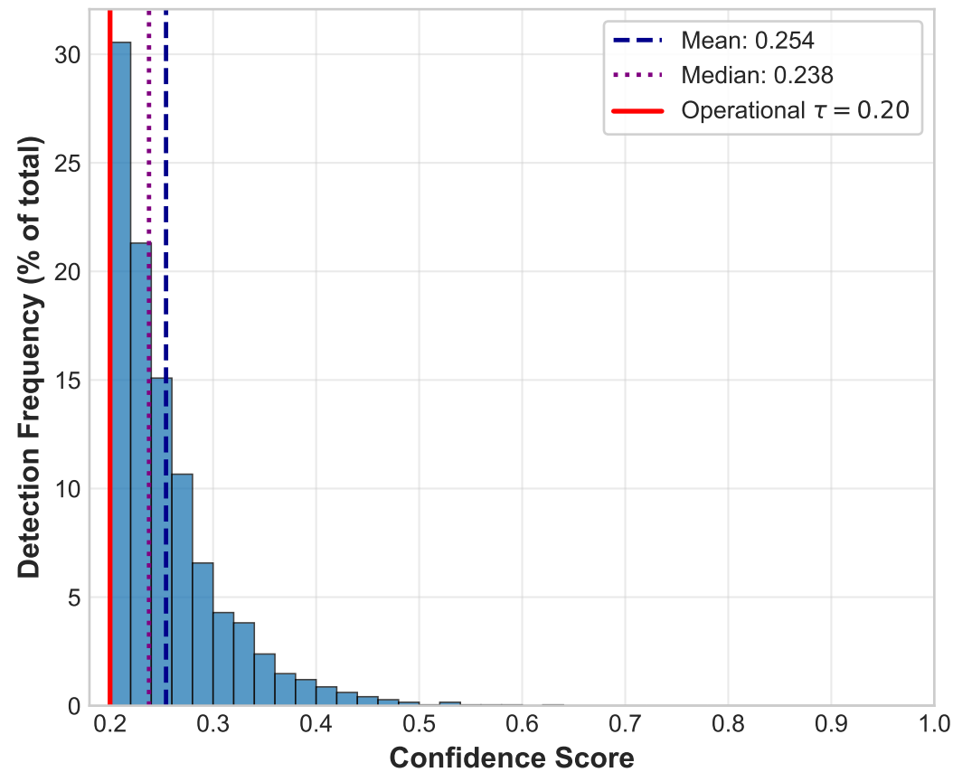
YOLO26n (N = 5,084)
