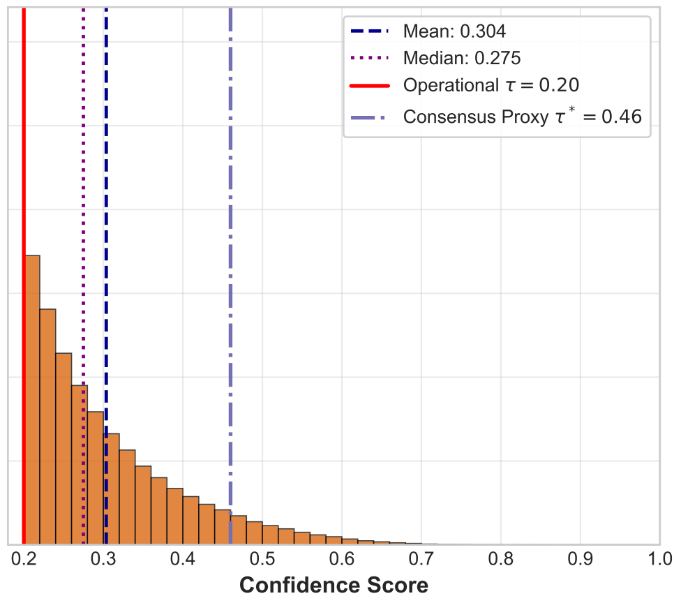
YOLOv8n (N = 353,427)
