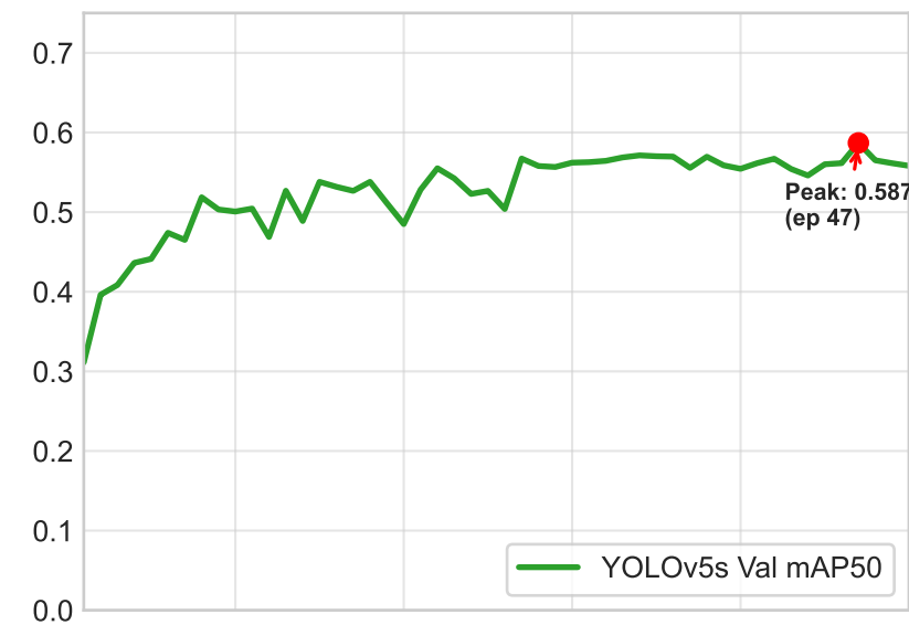
YOLOv5s
