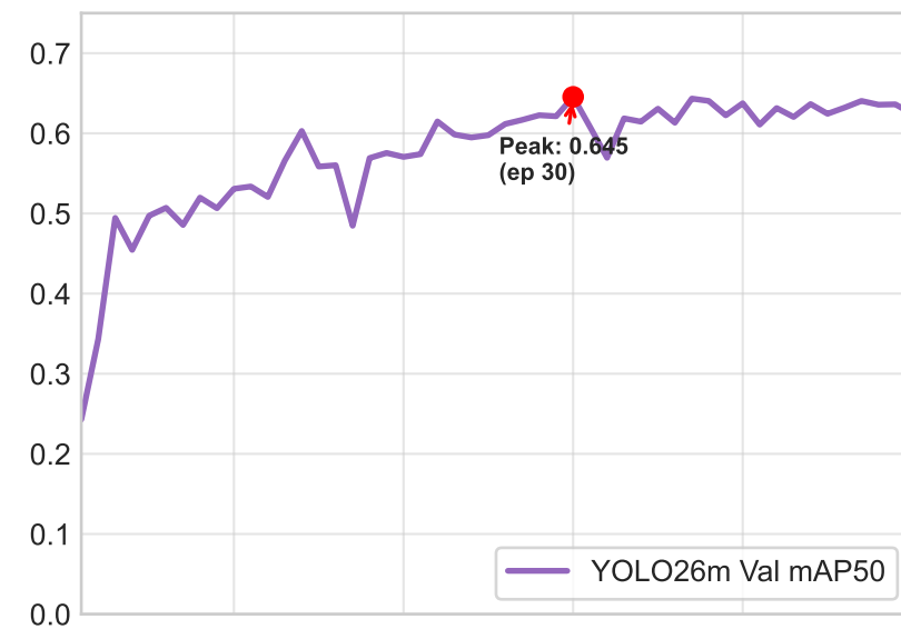
YOLO26m
