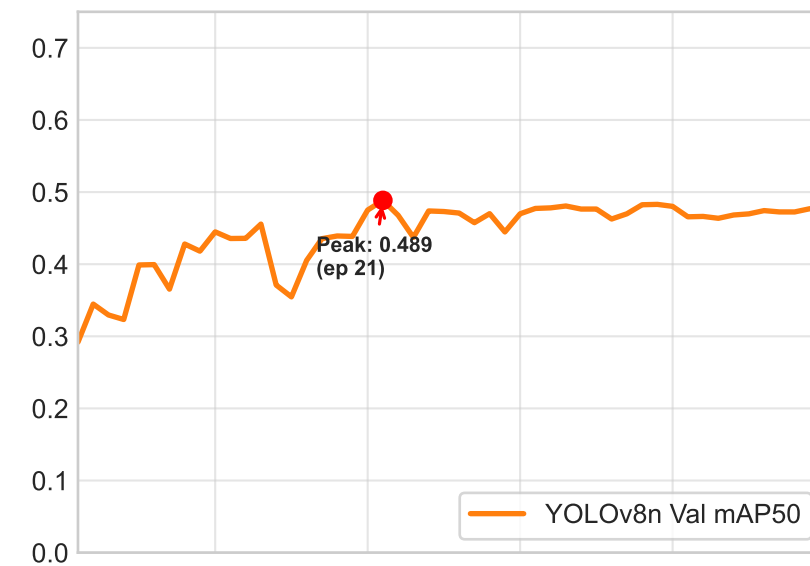
YOLOv8n
