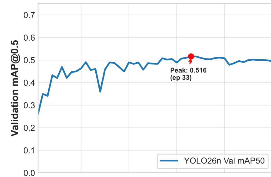
YOLO26n
