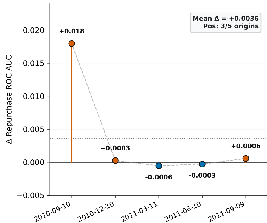
(d) Online Retail II · \Delta Repurchase ROC AUC
