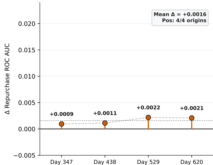
(d) Online Retail II · \Delta Repurchase ROC AUC
