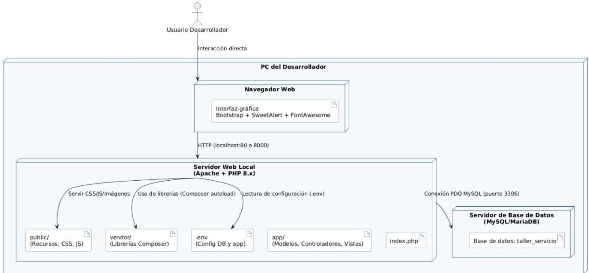
Diagrama de Despliegue - Entorno Local (Apache + PHP + MySQL)
