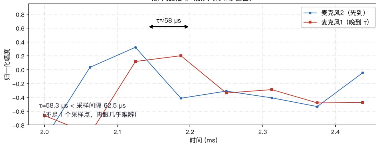
图12 GCC-PHAT 声源定位原理：亚采样时延估计（模拟）
