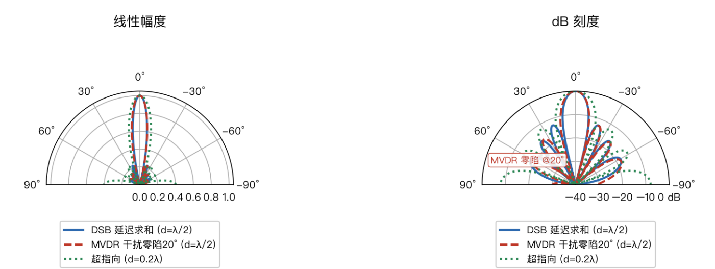
图16 8元ULA 0°指向波束图对比：DSB / MVDR(零陷@20°) / 超指向 (f=2kHz, d=λ/2, c=343m/s, 上=0°正横, 模拟)
