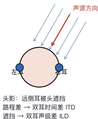
(b) 双耳时间差 ITD (Woodworth 模型)
