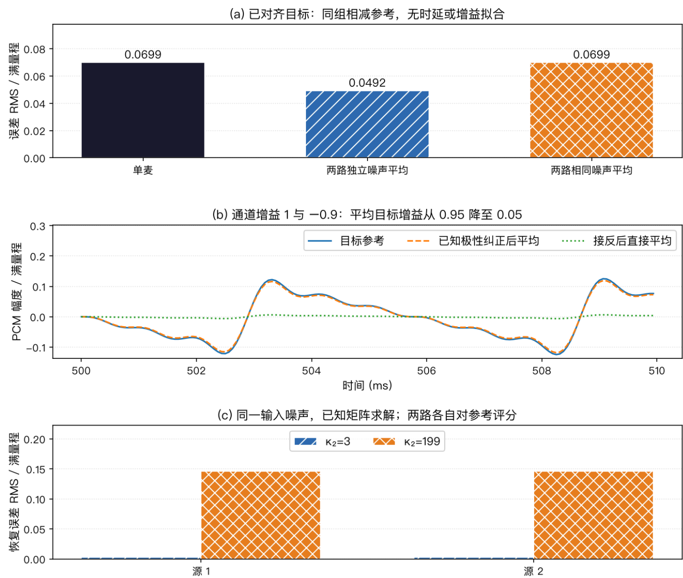
图 35 读取 16 kHz、PCM16 导出文件，每组使用共同增益，随机种子 20260923，时长 2 s。(a) 两路目标已对齐，噪声标准差均为 0.07；独立噪声平均后误差 RMS 下降，复制相同噪声则不下
