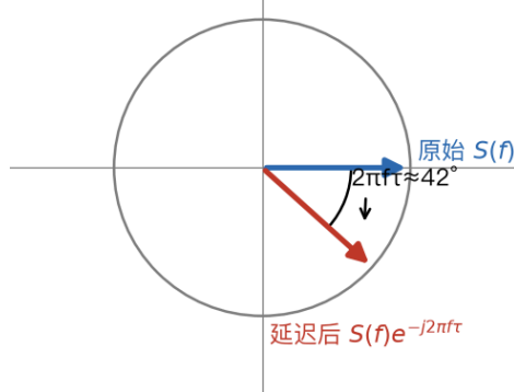
(b) 频域看延迟：复数相位转过一个角度 延迟 \tau 等价于复平面上 顺时针转 2\pi f\tau
