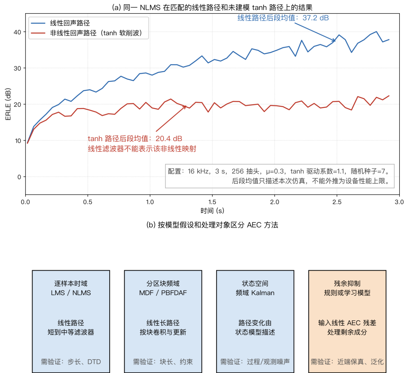
图19 AEC 的模型失配与方法分类
