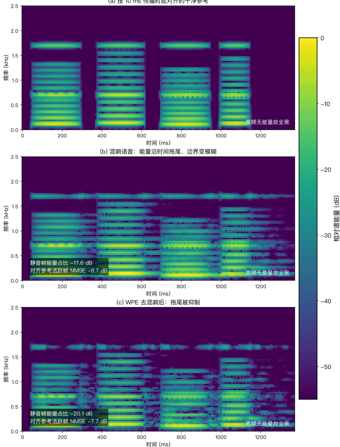
图21 WPE 去混响效果（本书单通道仿真）
