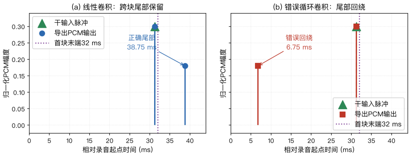
图49 同一脉冲与稀疏121抽头FIR的块边界（最终PCM读回）
