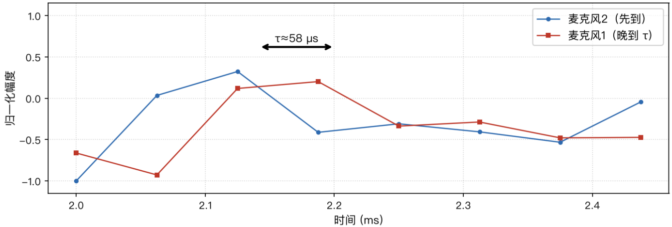
(a) 两路信号（放大 0.5 ms 窗口）
