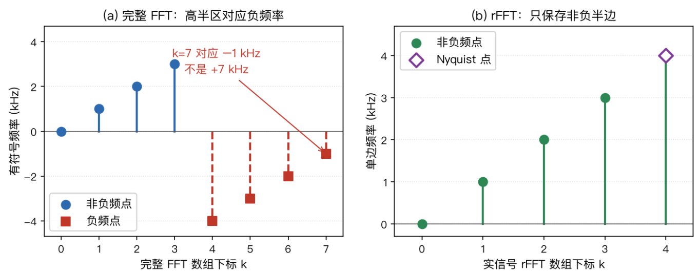
图48 N=8、采样率8 kHz的两种频点标记
