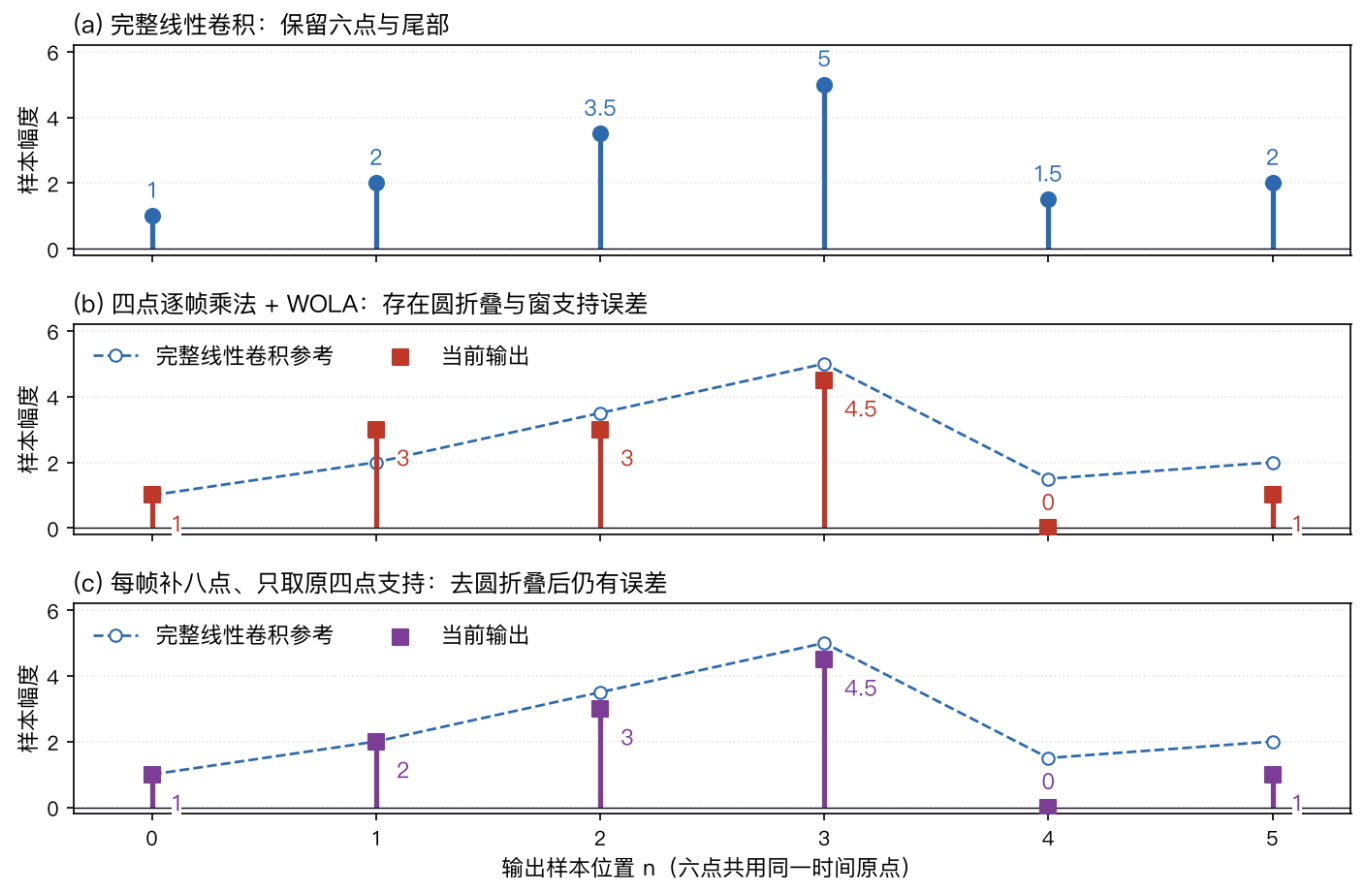
图50 有限窗的逐帧乘法为何不等于完整卷积
