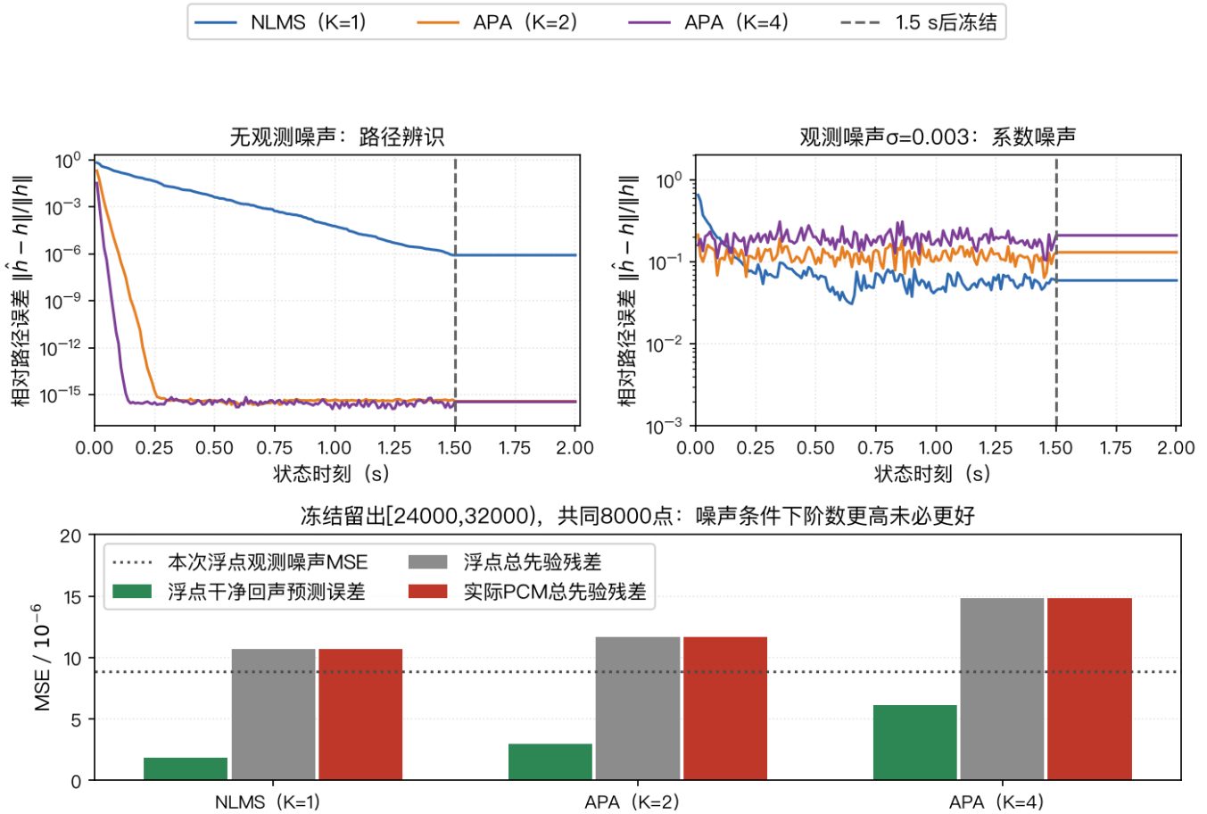
图58 有色参考下的收敛与噪声代价
