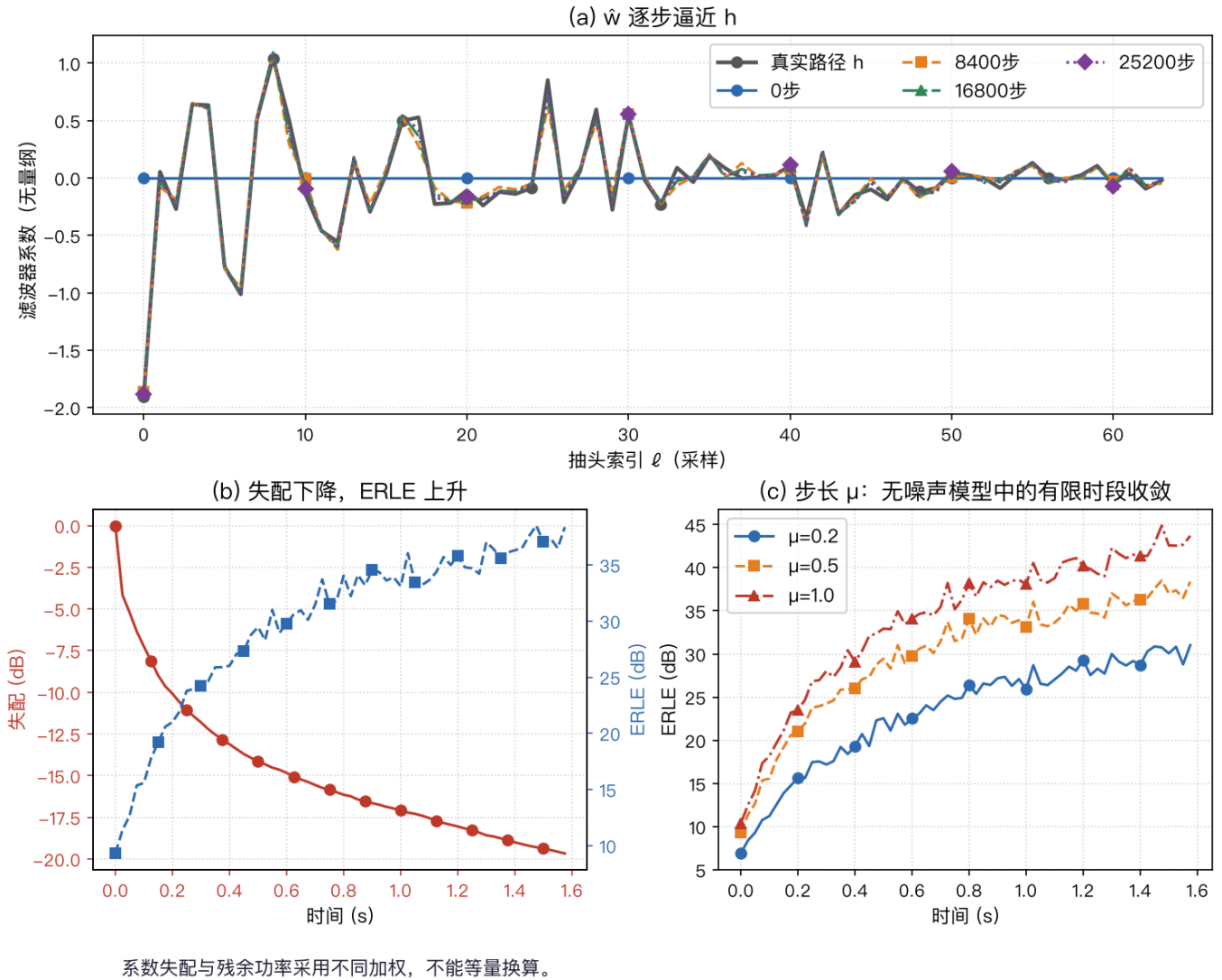
图28 NLMS 自适应：路径估计逐步逼近真实响应
