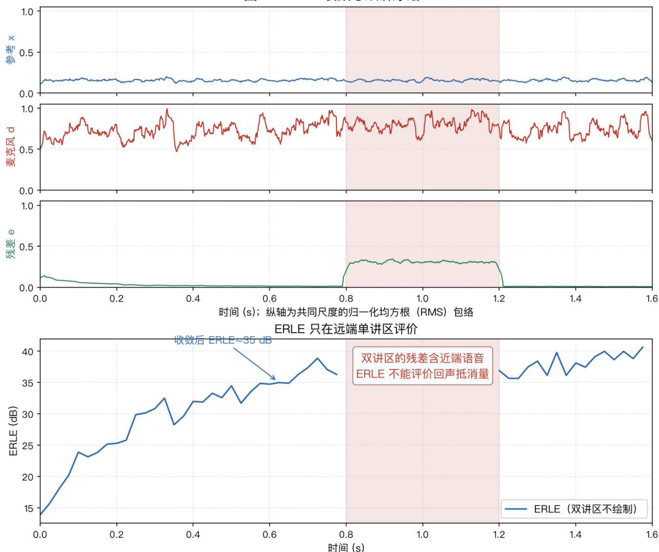
图29 NLMS 收敛与双讲冻结
