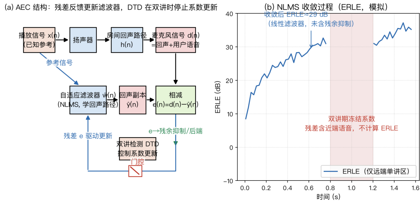
图18 (a) 给出整体结构；(b) 给出 NLMS 在模拟回声路径上的收敛曲线。仿真取 \mu = 0.5 ，回归向量按 \vec{x}(n) = [x(n), x(n - 1), \dots, x(n - L + 1)]^\top 排列，与生成回声的卷积索引一致，不额外引入一拍延迟。图中标注的是固定随机种子下 0.45 < t < 0.8 s 远端单讲窗口的 ERLE 均值；粉色区域表示双讲期间冻结更新，该区间不统计 ERLE。
