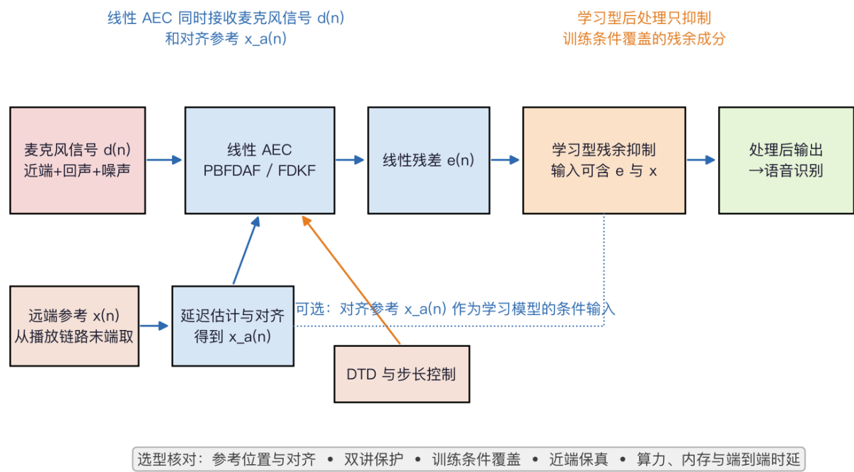
图32 线性回声消除与残余抑制：按系统条件选择模块 混合处理流程：线性前级与残余后处理各有适用前提
