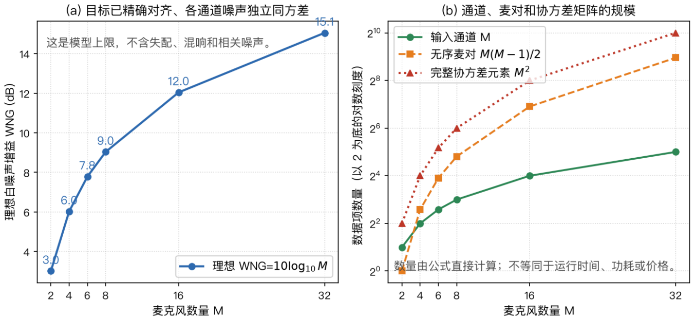
图9 麦克风数量增加时的理想增益与处理量 (公式计算，不给出产品选型排名)
