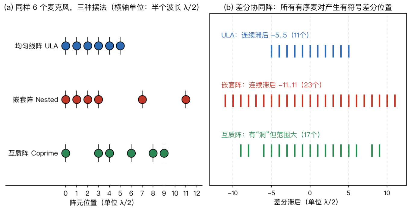
图 10 左侧比较均匀、嵌套和互质三种摆法，横轴单位是半波长；右侧枚举所有有序麦对的位置差，得到有符号差分位置（也称有符号滞后）。均匀阵有 11 个连续滞后，图中的嵌套阵有 23 个连续滞后，互质阵覆盖范围更大但中间有空缺。连续滞后数描述虚拟孔径结构，不应直接写成 MUSIC 可分辨的源数。
