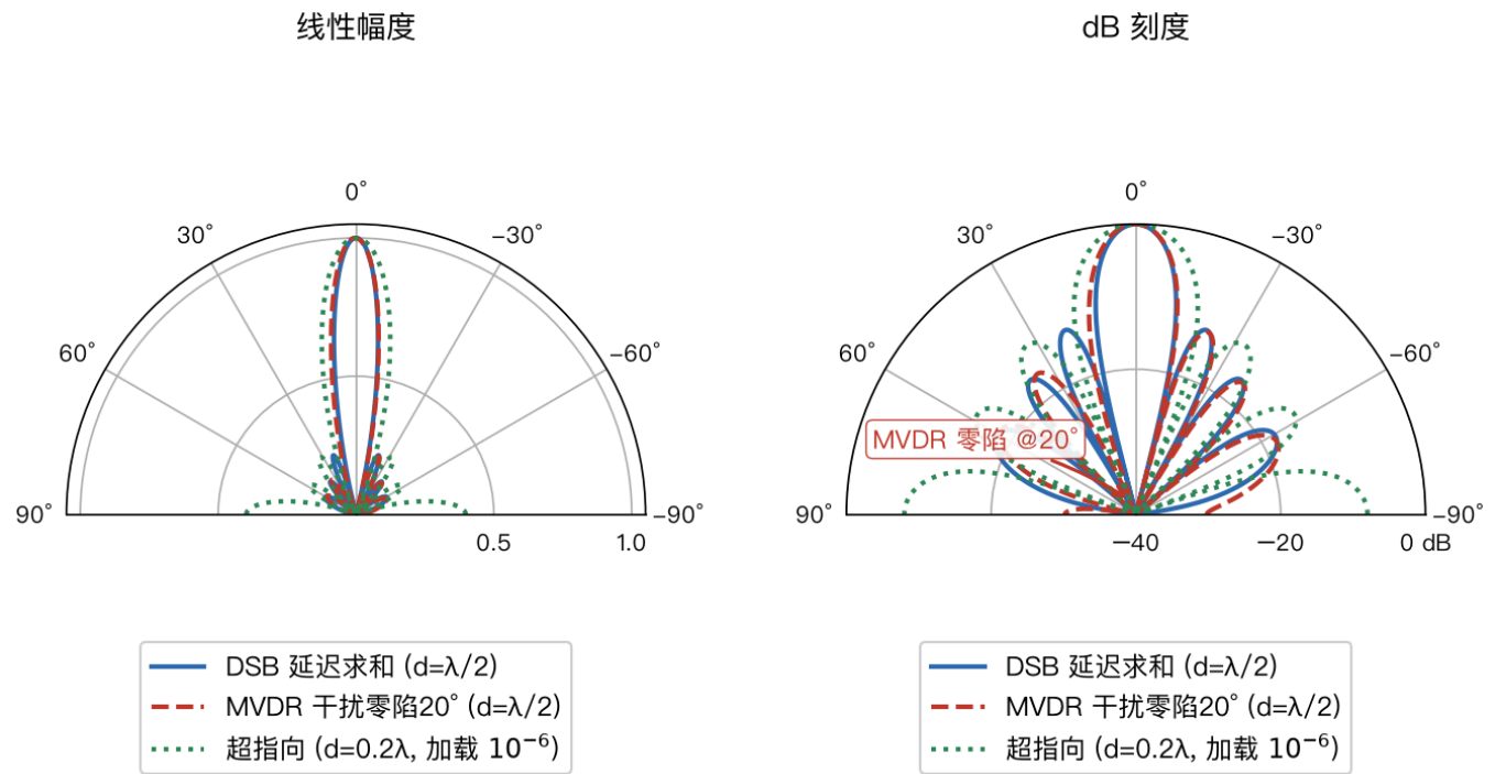
图16 8元ULA 0^\circ 指向波束图: DSB/MVDR 用 d=\lambda/2 , 超指向用 d=0.2\lambda (各曲线保持目标方向单位响应; MVDR 干扰=20°; 超指向相对对角加载=10 -6 ; 模拟)
