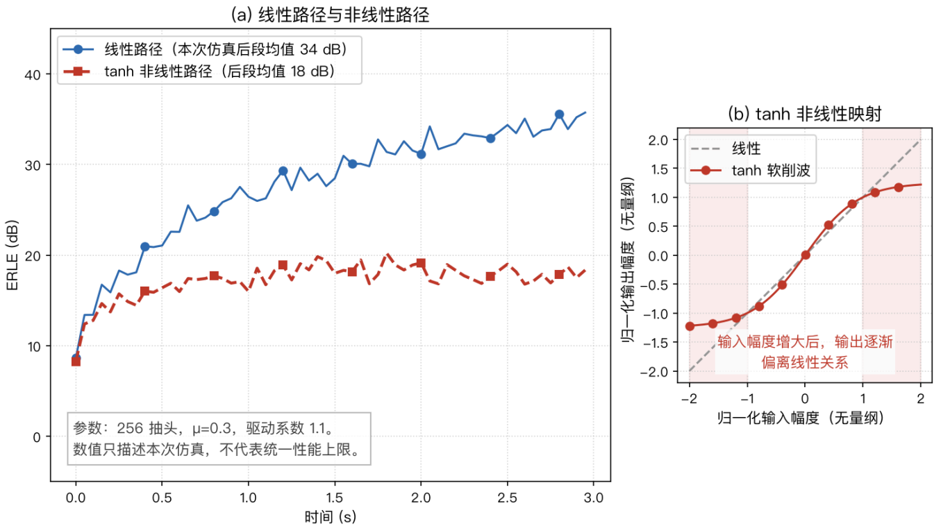
图31 本仿真中的线性匹配与非线性失配
