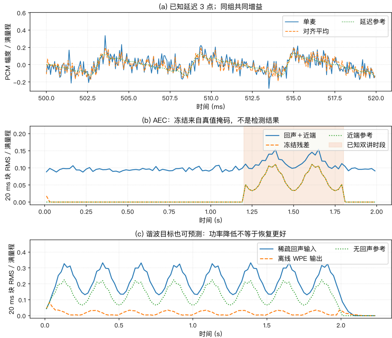
图 34 直接读取已导出的 PCM：(a) 在 500~520 ms 对比晚到 3 个采样的参考、单麦与对齐平均；(b) 用 20 ms 块 RMS 标出 1.2~1.8 s 的已知双讲冻结；(c) 对比含 40 ms、80 ms 副本的输入、离线 WPE 和无回声参考。三组均为 16 kHz 合成信号，每组共用导出增益，不作单文件峰值归一化。
