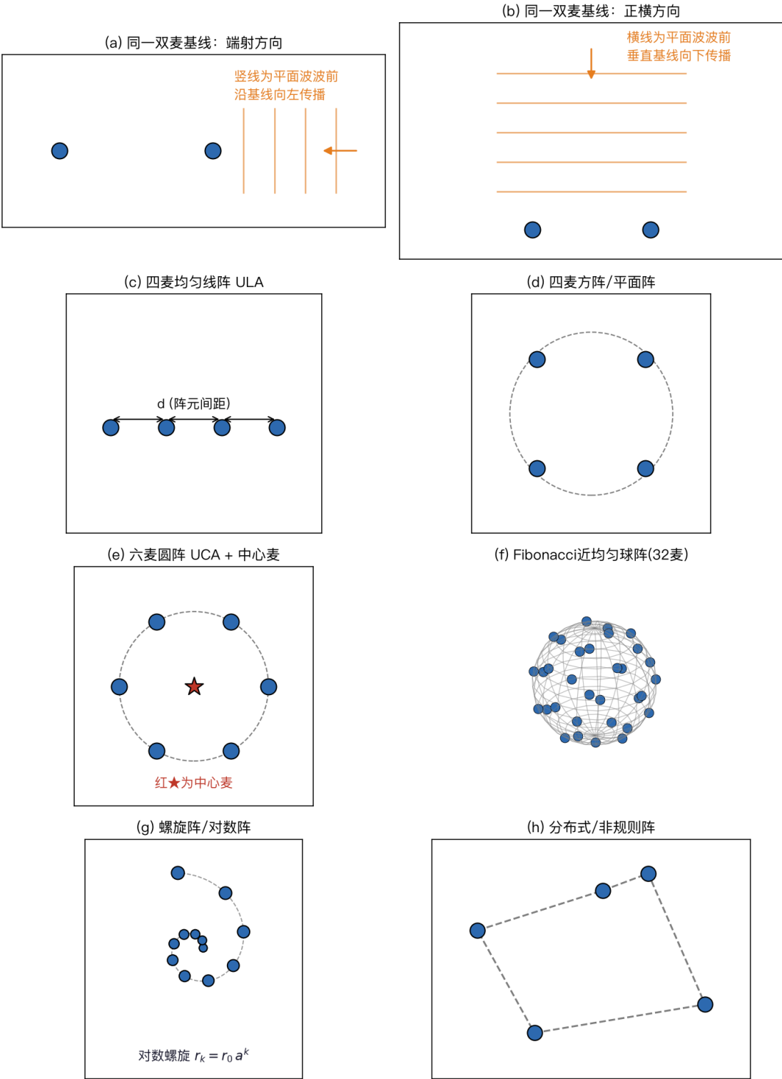
图8 常见麦克风阵列几何形态示意
