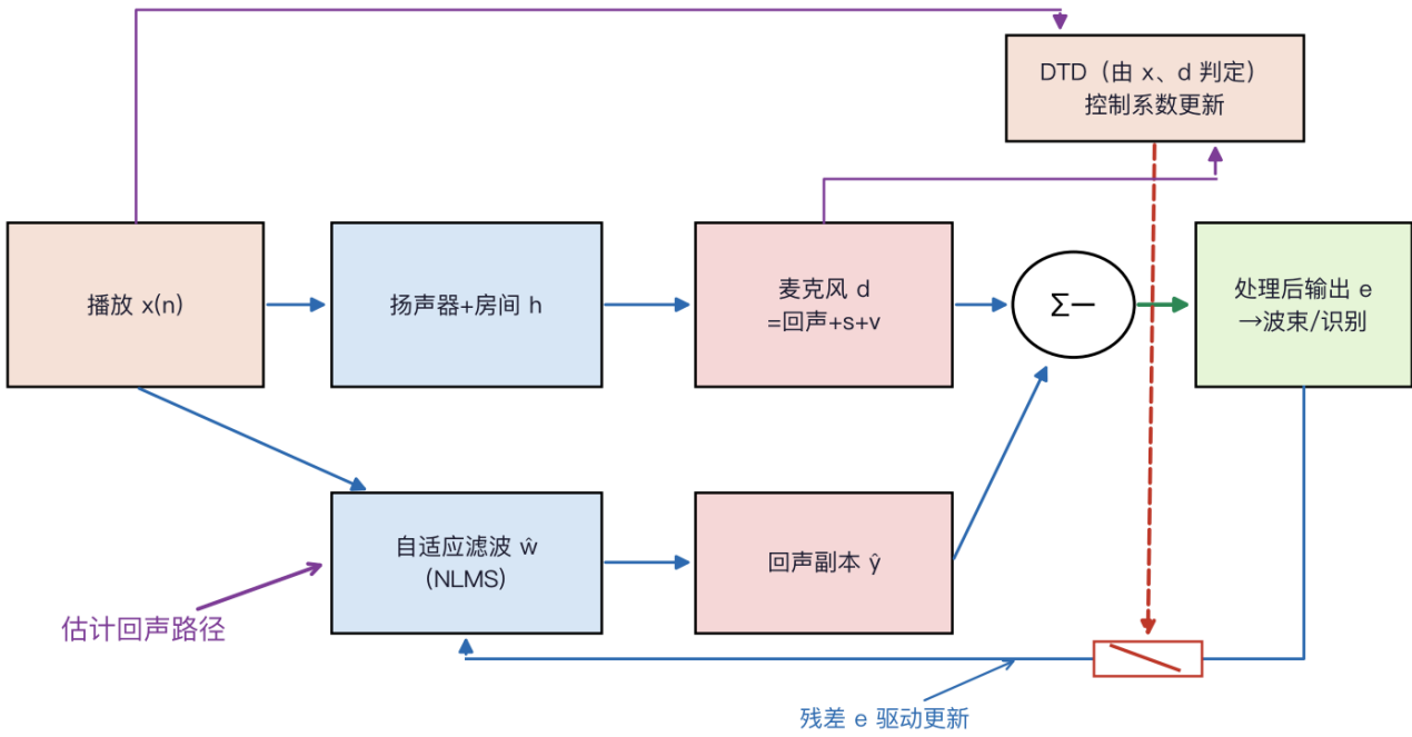
图27 AEC 结构：根据播放参考估计回声，再从麦克风信号中相减
