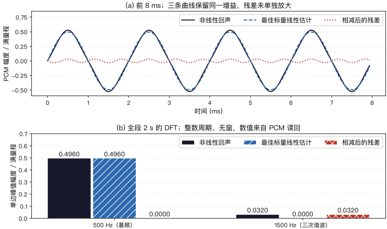
图36 三次非线性留下线性估计无法表示的谐波（合成反例）
