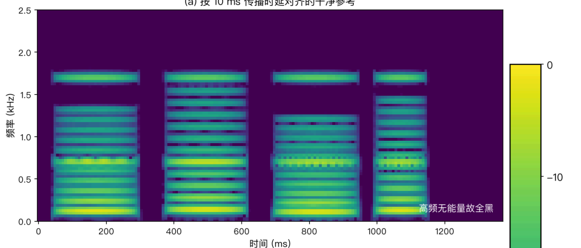
图21 WPE 去混响效果（本书单通道仿真）
