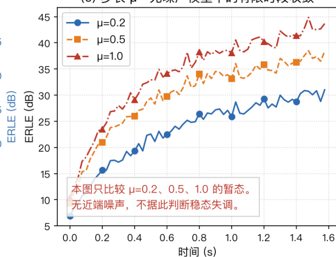
(c) 步长 \mu : 无噪声模型中的有限时段收敛
