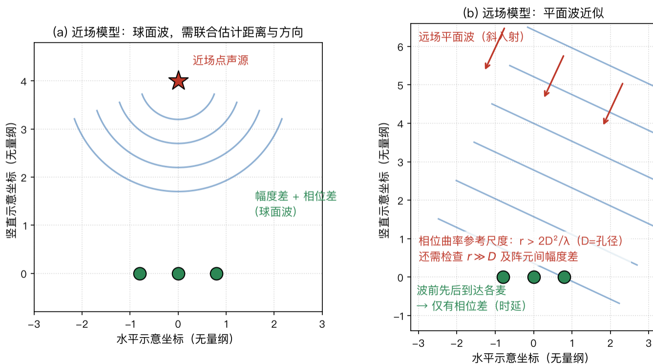
图3 近场与远场声场模型
