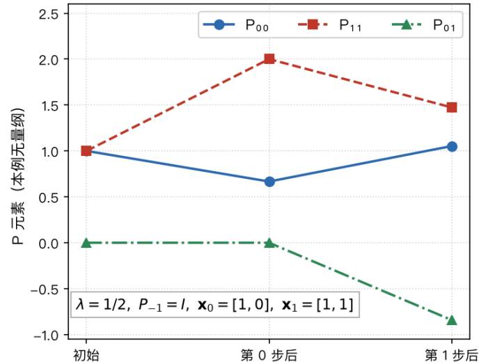
(b) RLS：P 是逆参考相关矩阵
