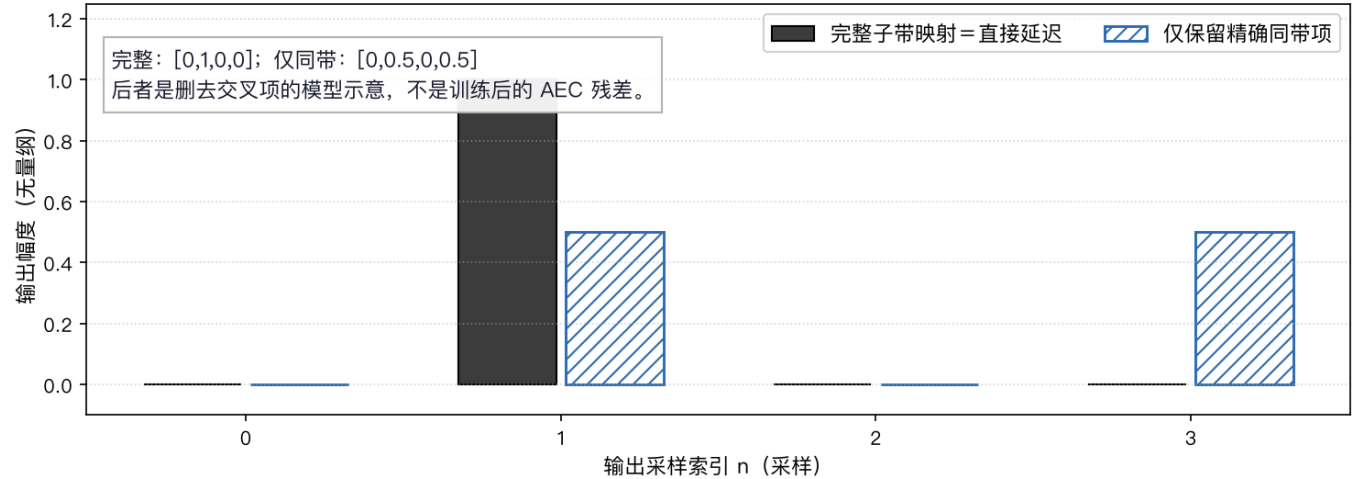
(b) 单位脉冲 x=[1,0,0,0] ，真实路径 y[n]=x[n-1]
