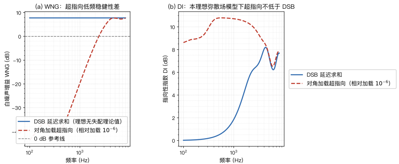
图15 6元圆阵（半径=相邻弦长=4 cm）超指向 vs 延迟求和：WNG与DI （三维各向同性弥散场；超指向相对对角加载= 10^{-6} ；目标方向单位响应；本书仿真）
