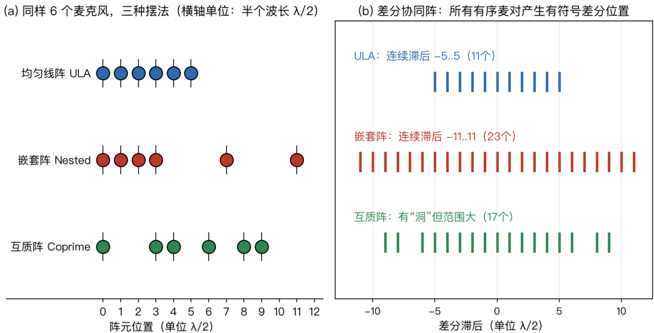
图10 稀疏阵列：6 个物理麦克风对应不同的有符号差分位置（模拟）
