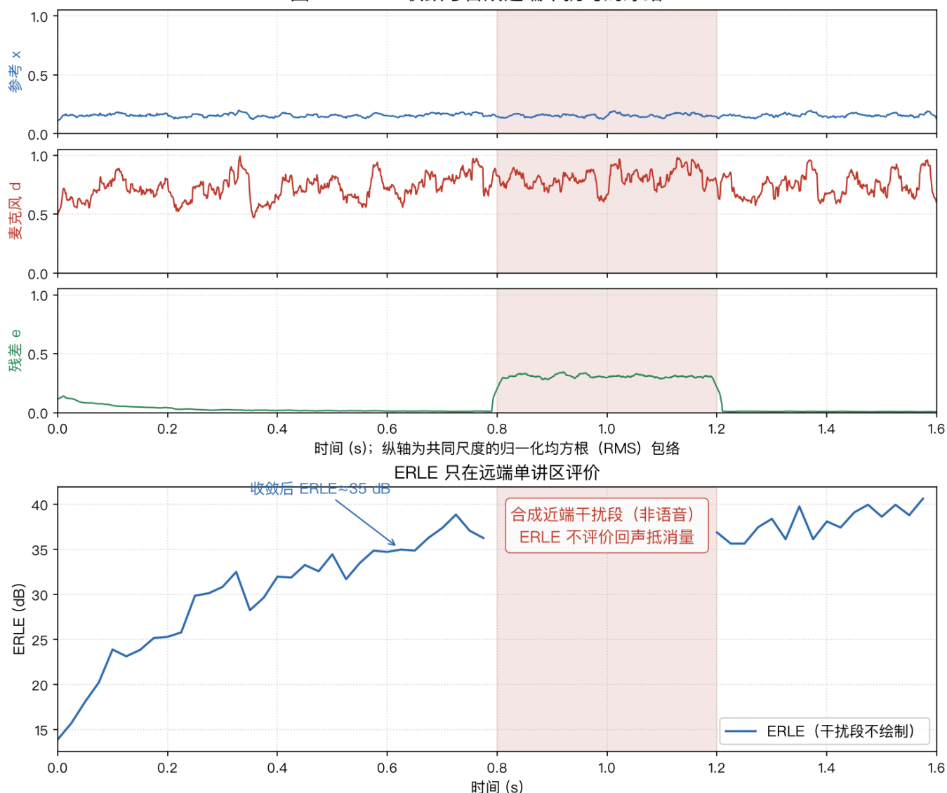
图29 NLMS 收敛与合成近端干扰时的冻结
