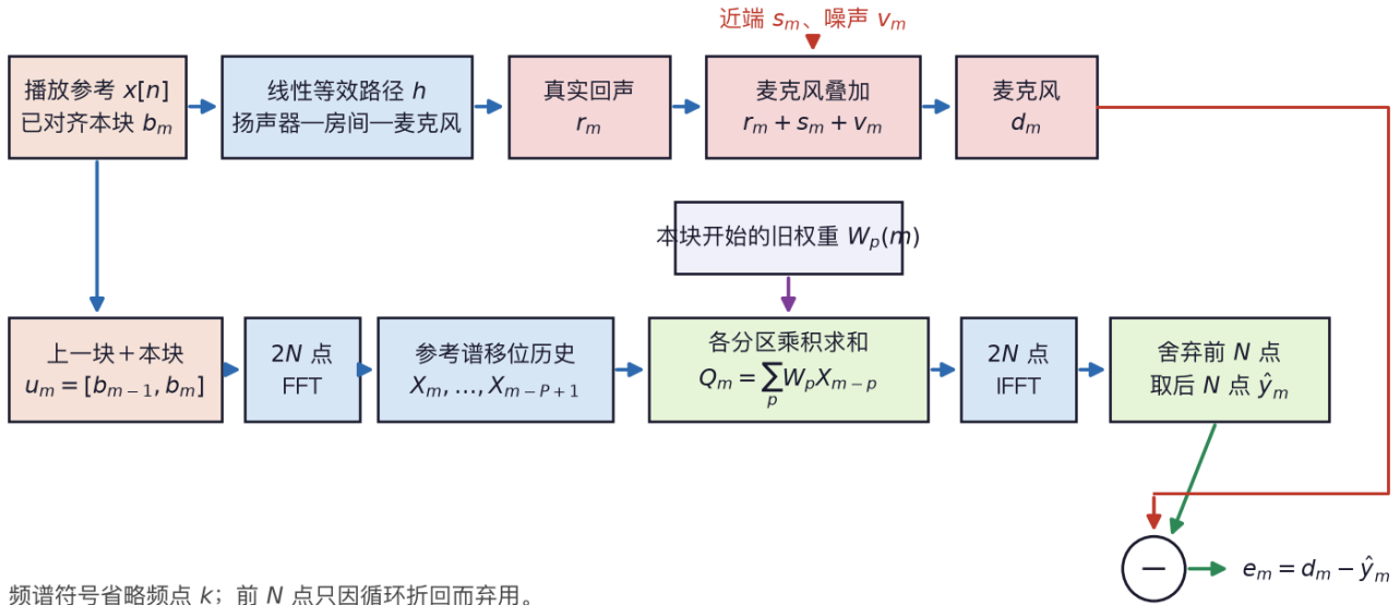
图39 PBFDAF：参考历史、有效输出与受控权重更新 (a) 旧权重先预测；仅循环卷积的后 N 点是本块有效输出
