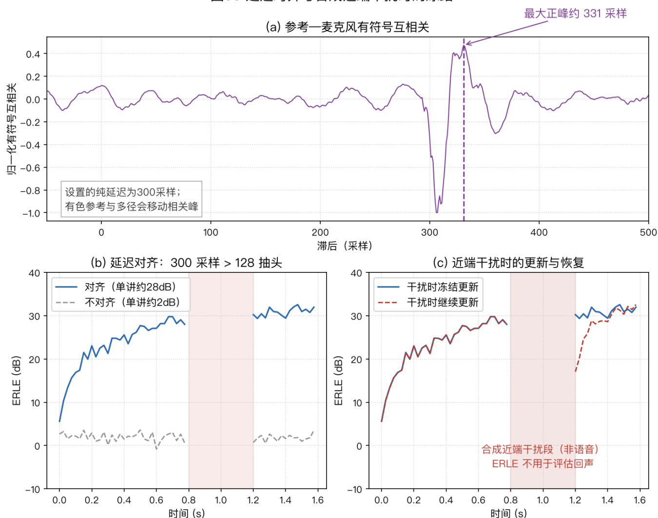
图30 延迟对齐与合成近端干扰时的冻结
