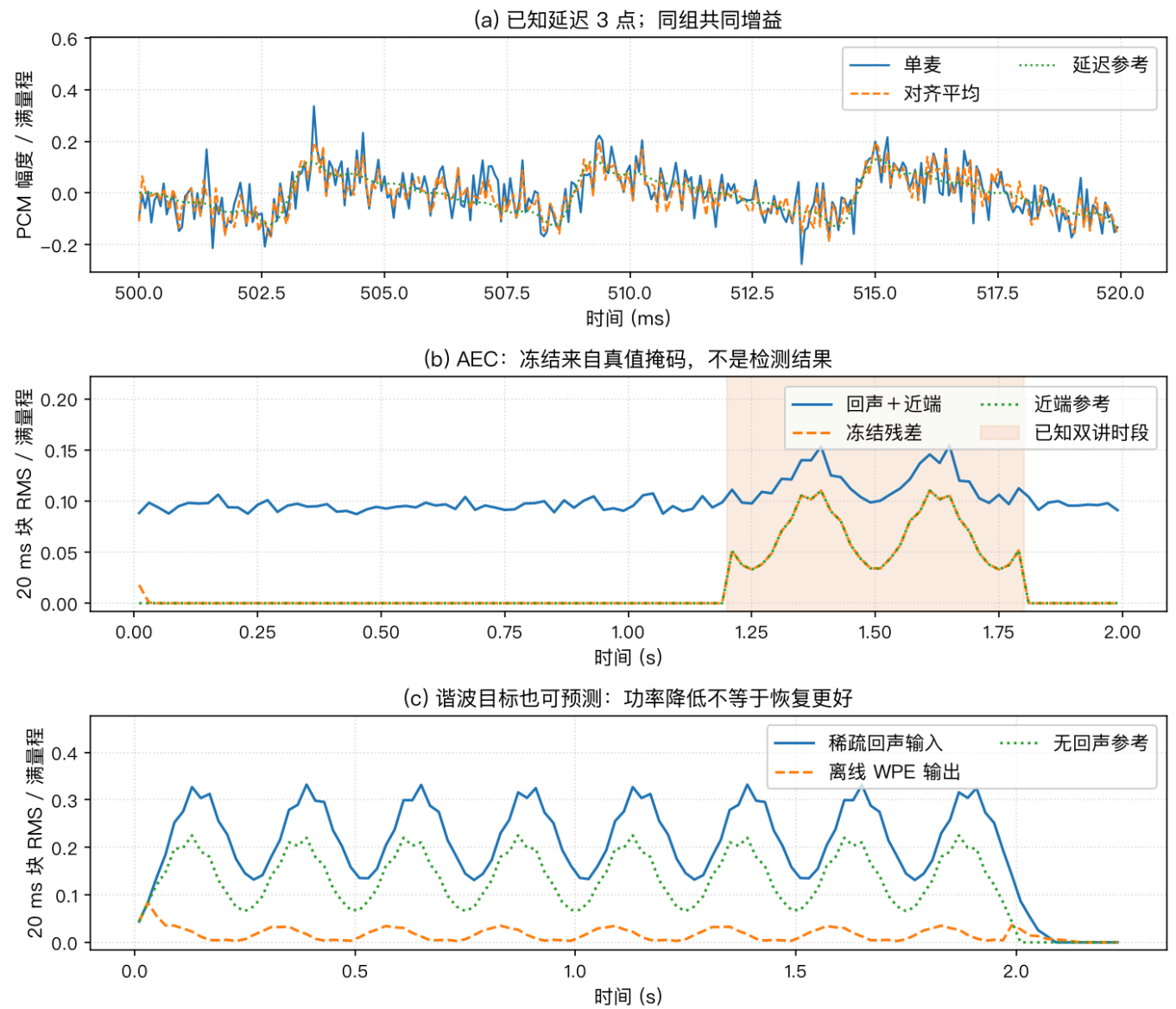
图 34 直接读取已导出的 PCM：(a) 在 500~520 ms 对比晚到 3 个采样的参考、单麦与对齐平均；(b) 用 20 ms 块的均方根（Root Mean Square，RMS）标出 1.2~1.8 s 的已知双讲冻结；(c) 对比含 40 ms、80 ms 副本的输入、离线 WPE 和无回声参考。三组均为 16 kHz 合成信号，每组共用导出增益，不作单文件峰值归一化。
