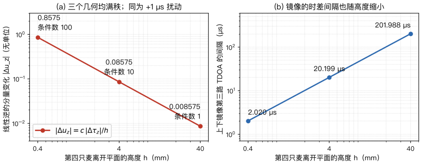
图51 满秩几何的线性敏感性与镜像时差
