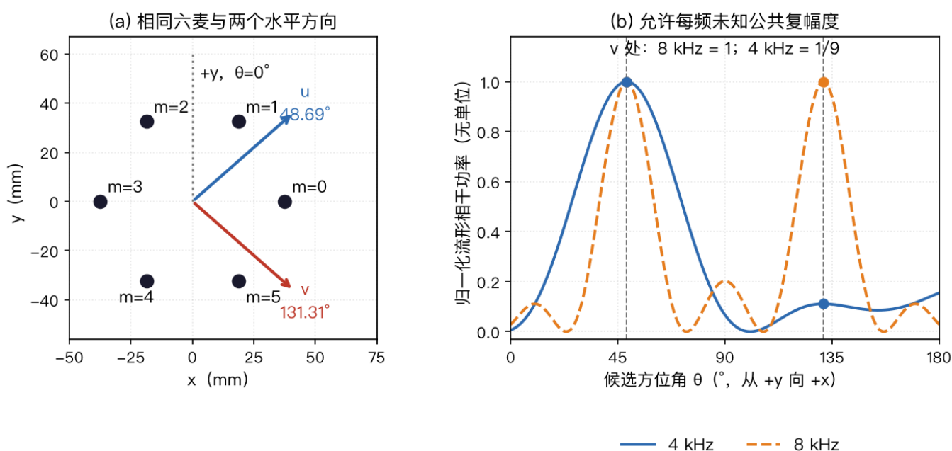
图52 第二个频率怎样区分单频别名
