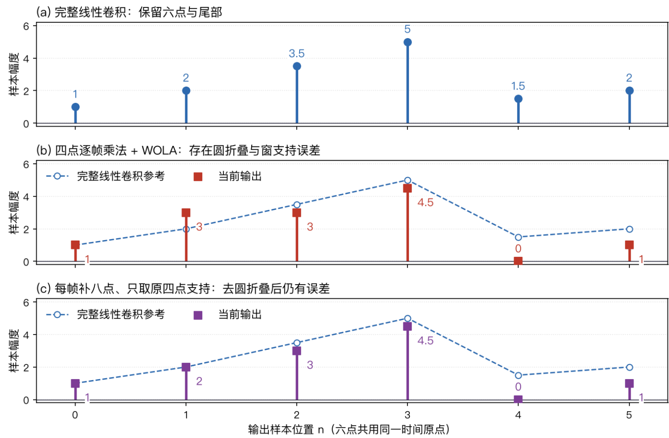
图50 有限窗的逐帧乘法为何不等于完整卷积
