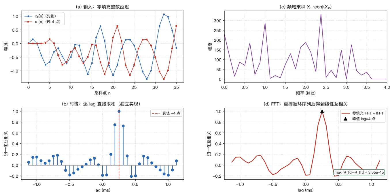
图33 互相关的两种等价实现 (GCC 中 \Phi(f)=1 的特例; 非 PHAT 加权)
