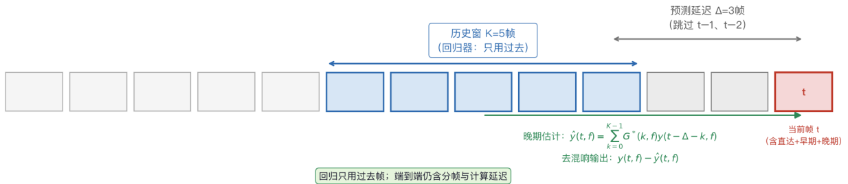
图24 WPE 延迟预测： \Delta=3 时保护 t-1 、 t-2 ， K=5 使用 t-3 \dots t-7
