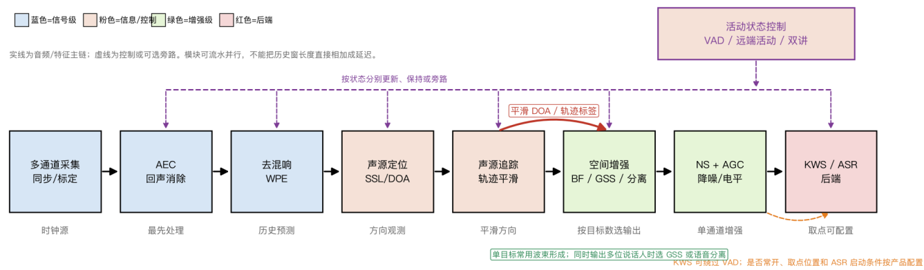
图23 远场语音前端：音频主链、方向反馈、状态控制与可选旁路
