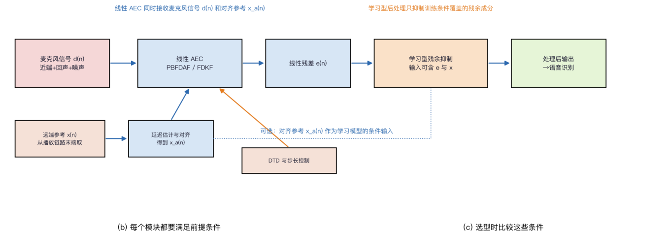
图32 线性回声消除与残余抑制：按系统条件选择模块 (a) 一种常见的混合处理流程
