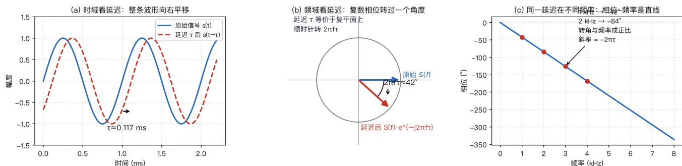
图4 时延为什么变成 e^{-j2\pi f\tau} ：几何直觉 (4 cm 麦距；端射方向达到最大麦间时延 \tau=d/c\approx 0.117 ms)
