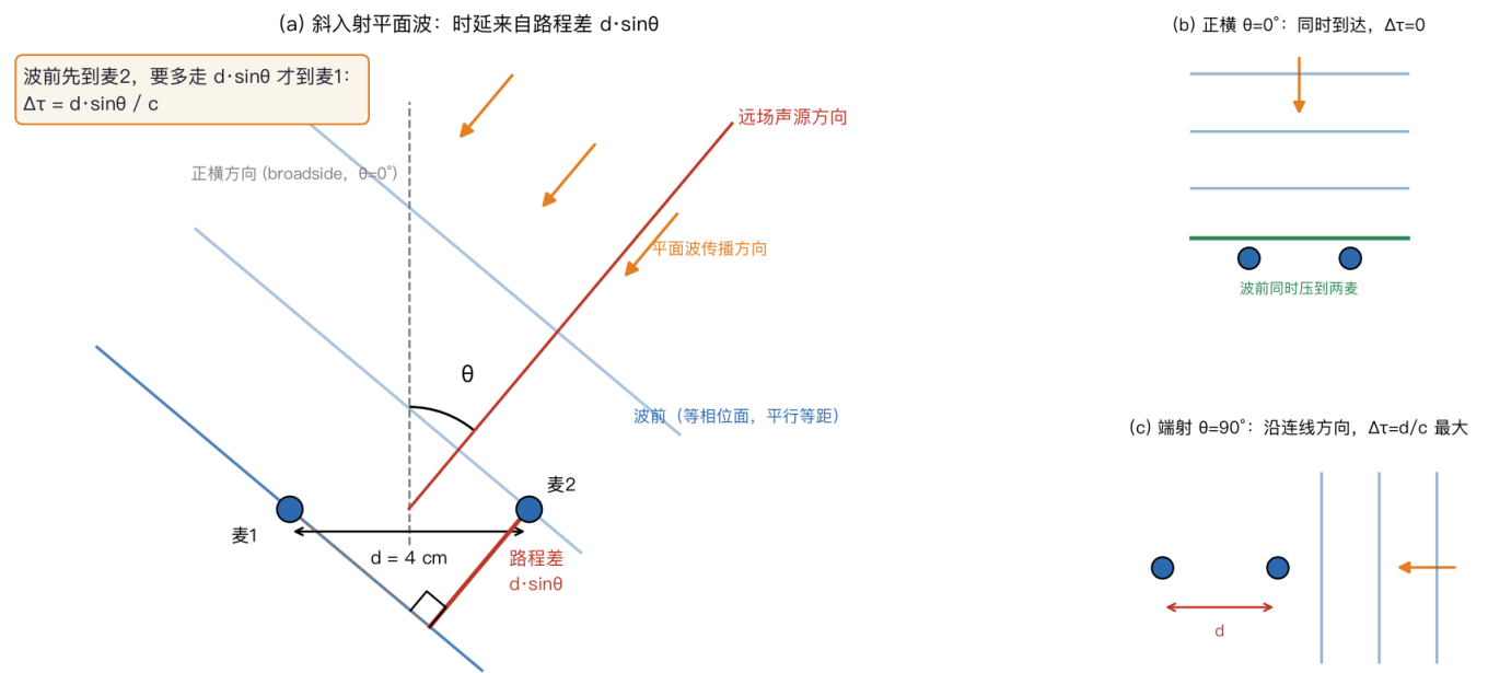
图2 时延的几何来源与角度约定（示意）
