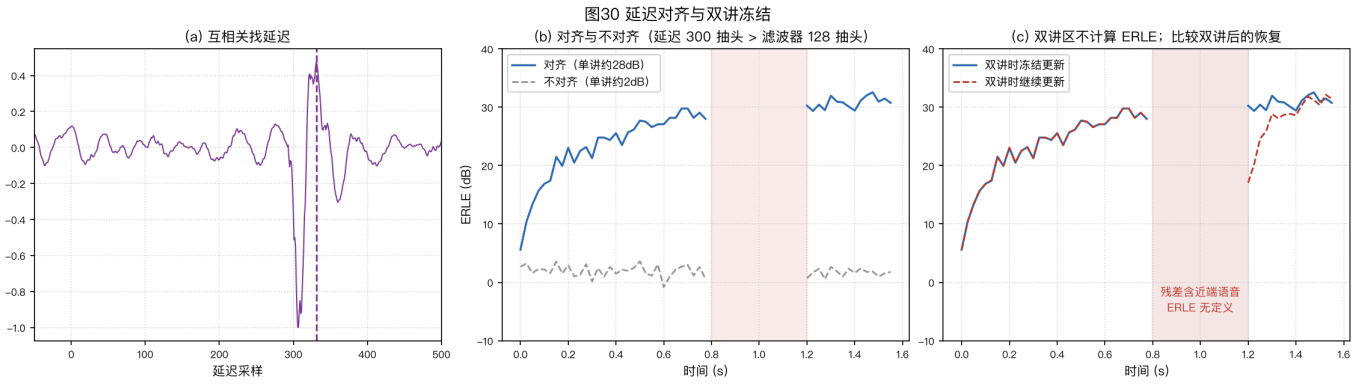
图30 (a) 用互相关估计参考与麦克风信号之间的延迟，本例峰值约为 331 个采样，其中包含设置的 300 个采样纯延迟和回声路径主峰的位置。(b) 对齐后的远端单讲 ERLE 约为 28 dB，不对齐时约为 2 dB。本例的纯延迟超过 128 抽头滤波器的覆盖范围，因此差异较大。(c) 比较双讲期间冻结和继续更新；后者会使路径估计偏离，双讲结束后需要重新收敛。排查时应分别检查延迟估计和双讲控制。
