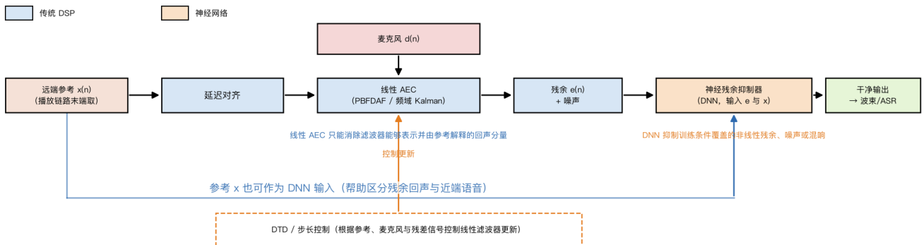
(b) 混合式处理链：线性回声估计 + 学习型残余抑制（示意）
