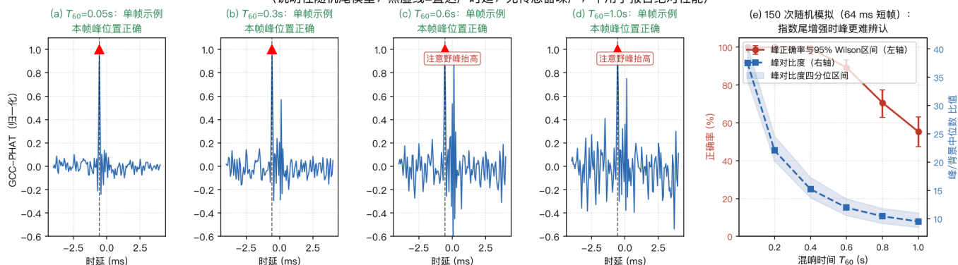
图13 随机衰减尾会扰乱 GCC-PHAT 峰 (说明性随机尾模型；黑虚线=直达声时延；无传感器噪声；不用于报告绝对性能)
