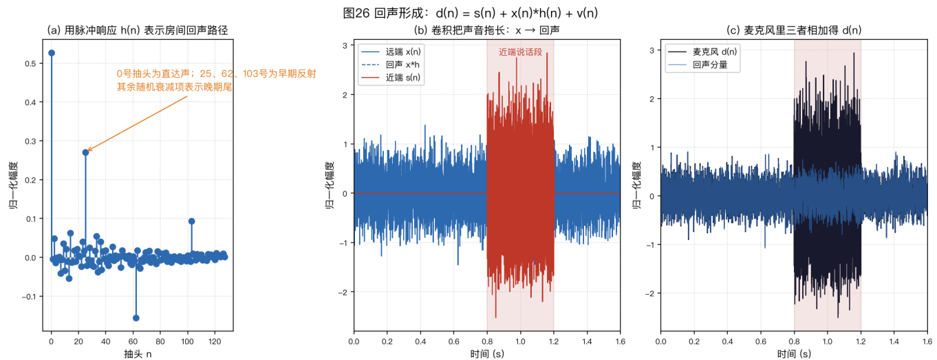
图26 (a) 的合成路径显式放置直达分量和若干早期反射，再叠加逐渐衰减的晚期尾声；这些成分只用于说明卷积结构，不代表某个实测房间。(b) 给出远端参考、卷积后的回声和 0.8~1.2 s 的近端语音。(c) 显示三者在麦克风信号 d(n) 中叠加。AEC 根据参考估计回声分量，再从 d(n) 中减去该估计。
