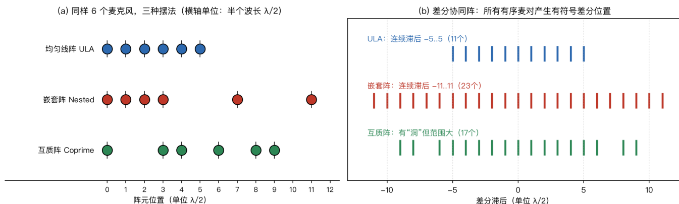
图10 稀疏阵列：6 个物理麦克风对应不同的有符号差分位置（模拟）
