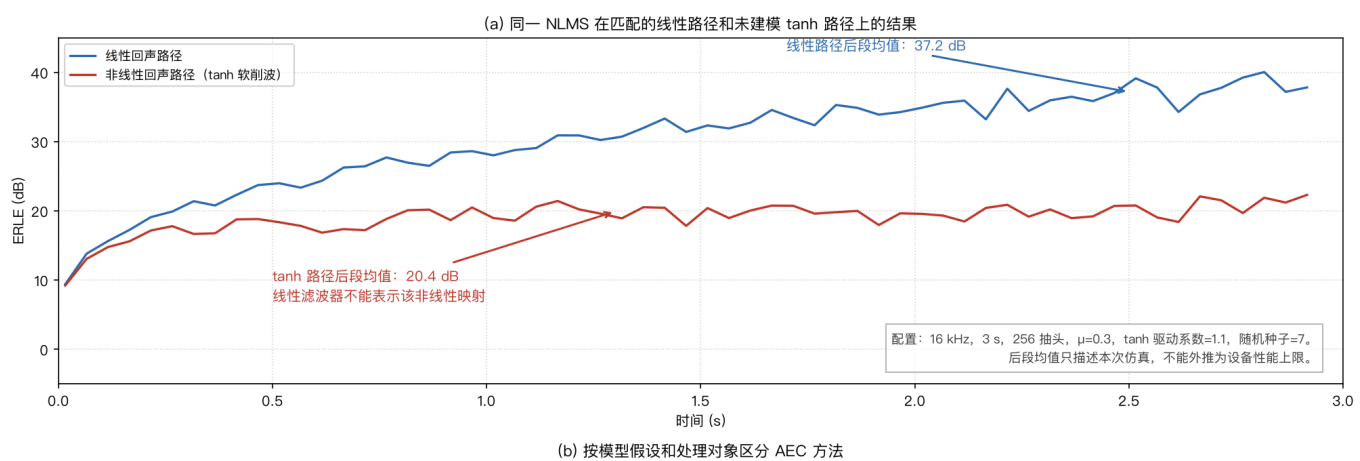
图19 AEC 的模型失配与方法分类
