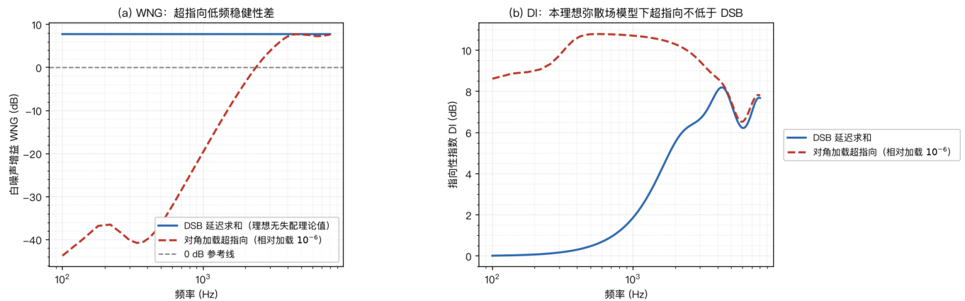
图15 6元圆阵（半径=相邻弦长=4 cm）超指向 vs 延迟求和：WNG与DI （三维各向同性弥散场；超指向相对对角加载= 10^{-6} ；目标方向单位响应；本书仿真）
