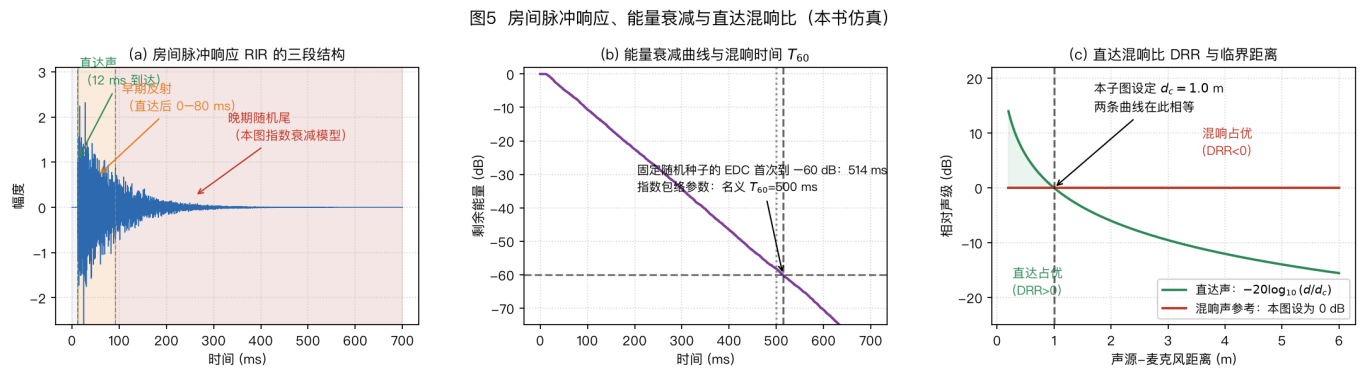
图 5 (a) 把房间脉冲响应分为直达声、早期反射和晚期混响；图 5 (b) 用能量衰减 60 dB 所需时间定义 T_{60} ；图 5 (c) 固定 d_c = 1.0 m，展示直达声与混响声的相对声级怎样随声源—麦克风距离变化。该子图是归一化示例，不直接给出体积或混响时间不同的房间结果。
