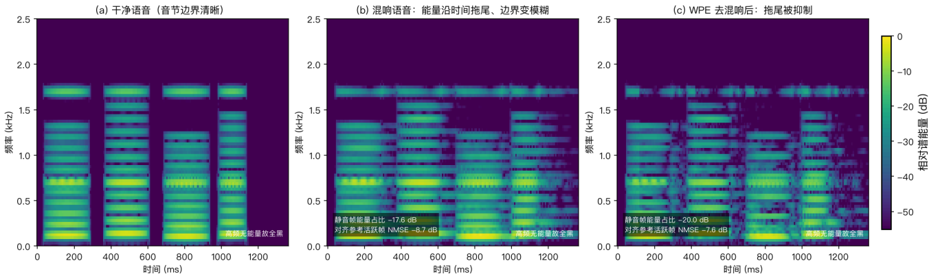
图21 WPE 去混响效果（本书单通道仿真）
