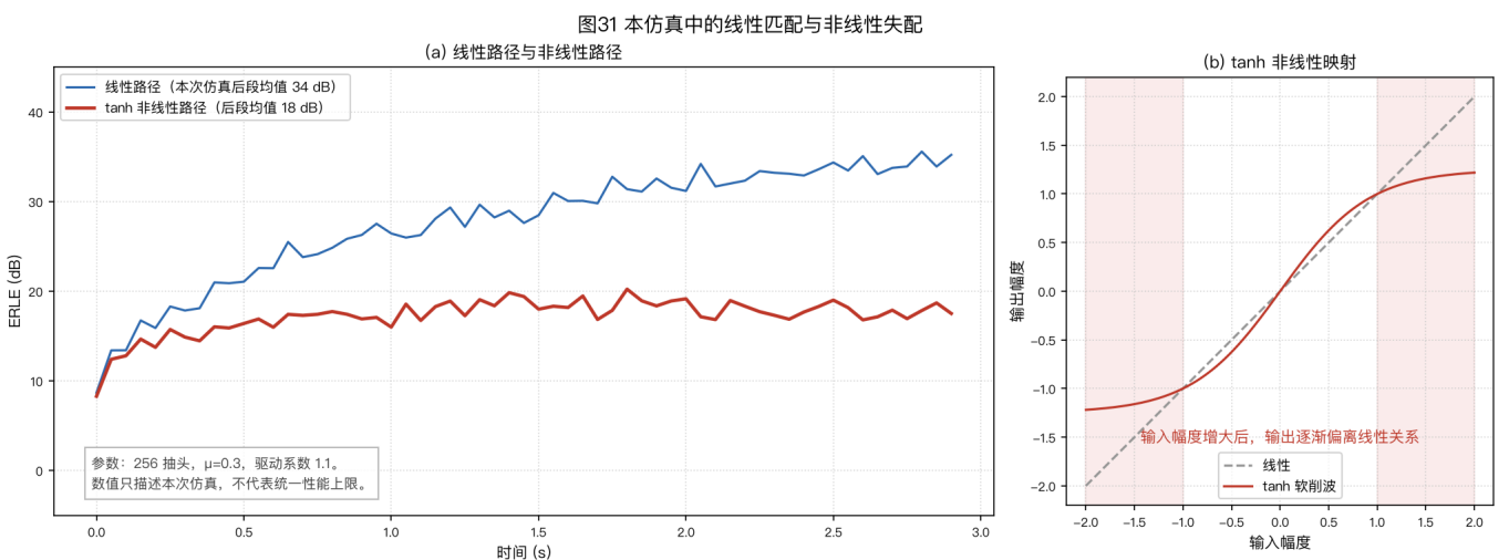
图31 (a) 在当前仿真参数下比较线性路径与 \tanh(1.1x)/\tanh(1.1) 非线性路径，后段均值由脚本按图示窗口计算，不是设备性能上限。(b) 显示同一映射相对参考直线 y = x 的曲率。线性滤波器无法精确表示由此产生的非线性分量，因此只增加抽头或调整步长不能消除该模型失配。
