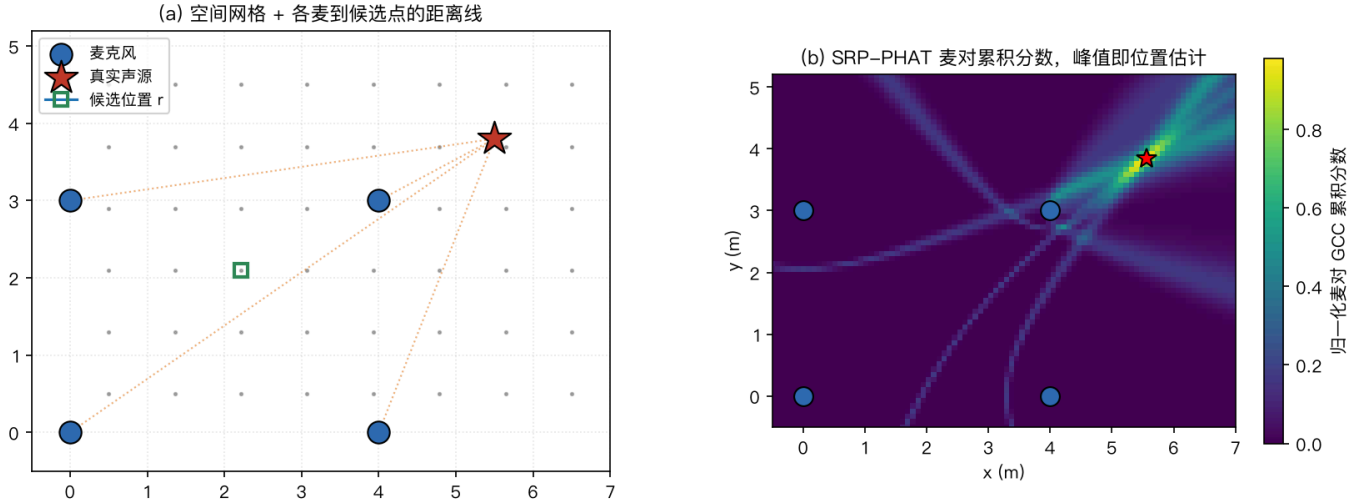
图14 SRP-PHAT 定位过程（理想化 GCC 峰；6 个麦对 TDOA 累积）
