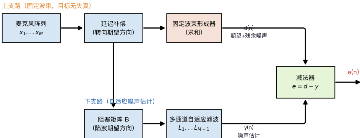
图17 GSC（广义旁瓣对消器）结构框图
