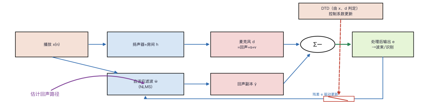
图27显示基本信号流：播放参考一支经过扬声器和房间进入麦克风，另一支进入自适应滤波器以估计回声路径。估计回声从麦克风信号中减去，双讲检测控制滤波器是否更新。
