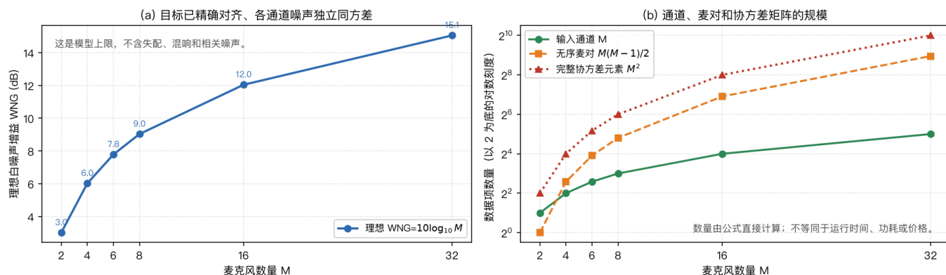
图9 麦克风数量增加时的理想增益与处理量 (公式计算，不给出产品选型排名)
