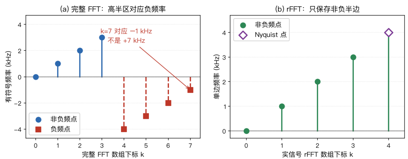
图48 N=8、采样率8 kHz的两种频点标记
