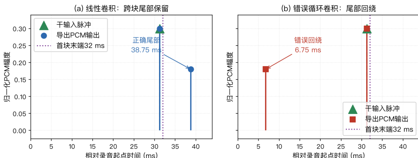
图49 同一脉冲与稀疏121抽头FIR的块边界（最终PCM读回）
