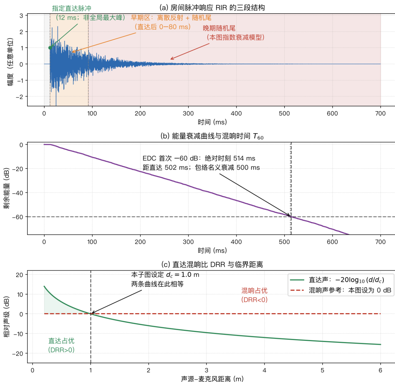
图5 房间脉冲响应、能量衰减与直达混响比（本书仿真）
