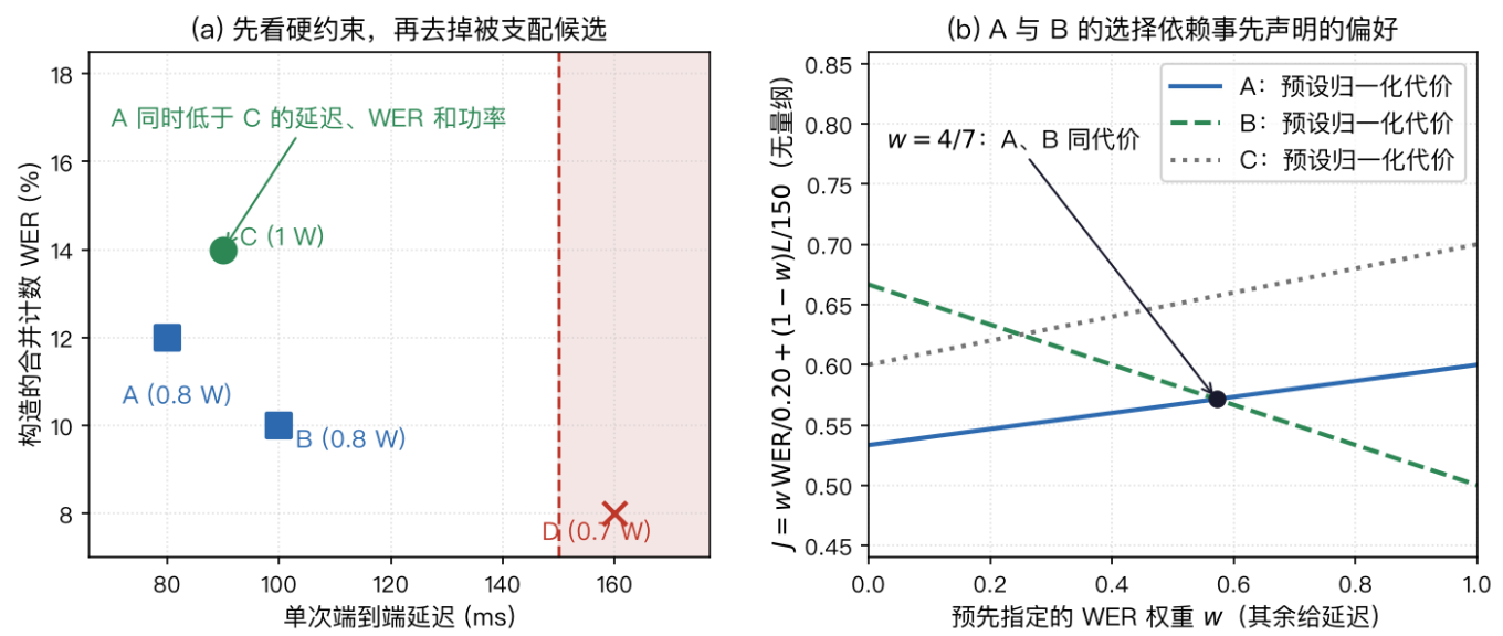
图 46: E11-10 的四个构造候选。(a) 横轴为延迟 (ms)，纵轴为 WER；功率分别为 A/B 0.8 W、C 1.0 W、D 0.7 W。先要求延迟不超过 150 ms、功率不超过 1 W，D 即使 WER 最低也不合格。合格集合中 A 支配 C，A 与 B 则各有优势。(b) 按式(11-4)比较 A/B 的归一化代价；质量权重 w = 4/7 时两者同分，权重变化会改变选择。图中的数值用于本书推导，不是四台设备的实测；(a) 的二维散点不能代替未画出的功率检查。
