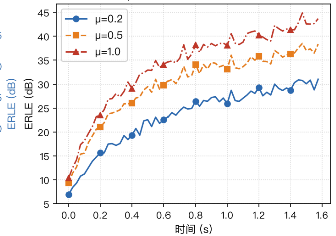
(c) 步长 \mu ：无噪声模型中的有限时段收敛
