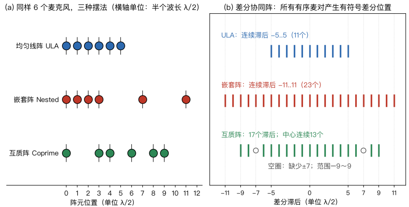
图10 六麦几何与有符号差分位置（按坐标枚举）
