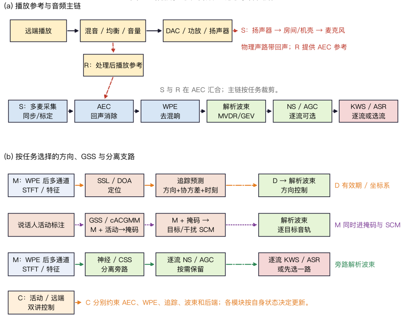
图23 播放参考、音频主链与条件支路
