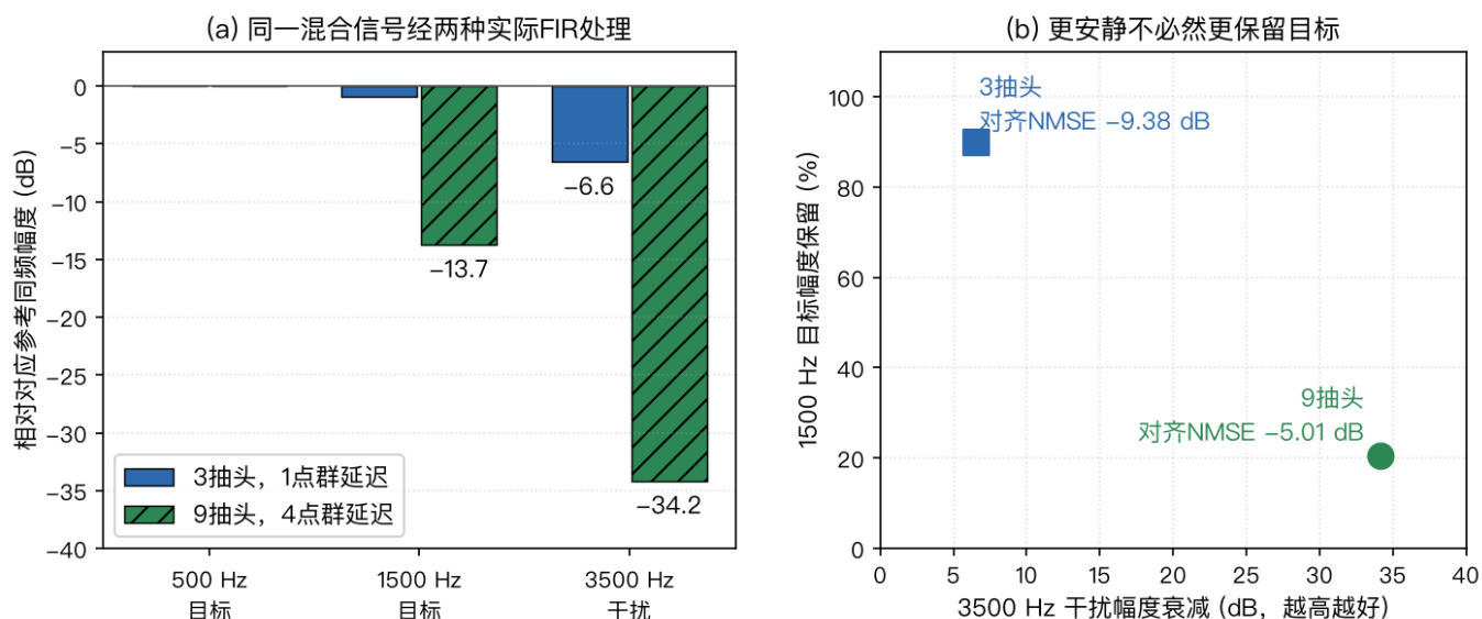
图47 固定三音合成输入的FIR选型取舍（最终PCM读回）
