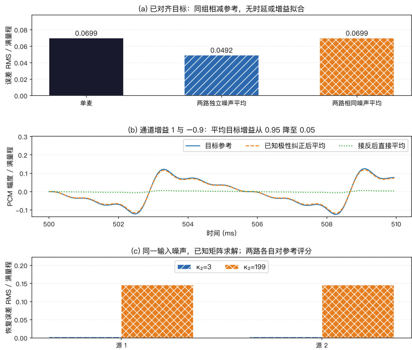
图 35 读取 16 kHz、PCM16 导出文件，每组使用共同增益，随机种子 20260923，时长 2 s。
