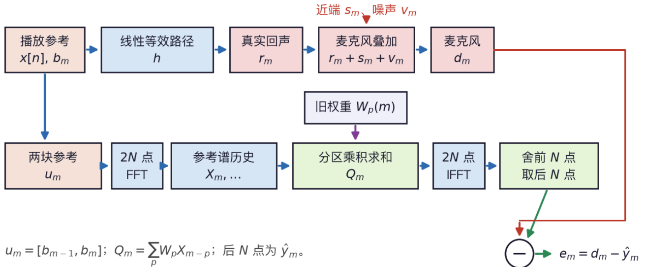
图39 PBFDAF：参考历史、有效输出与受控权重更新
