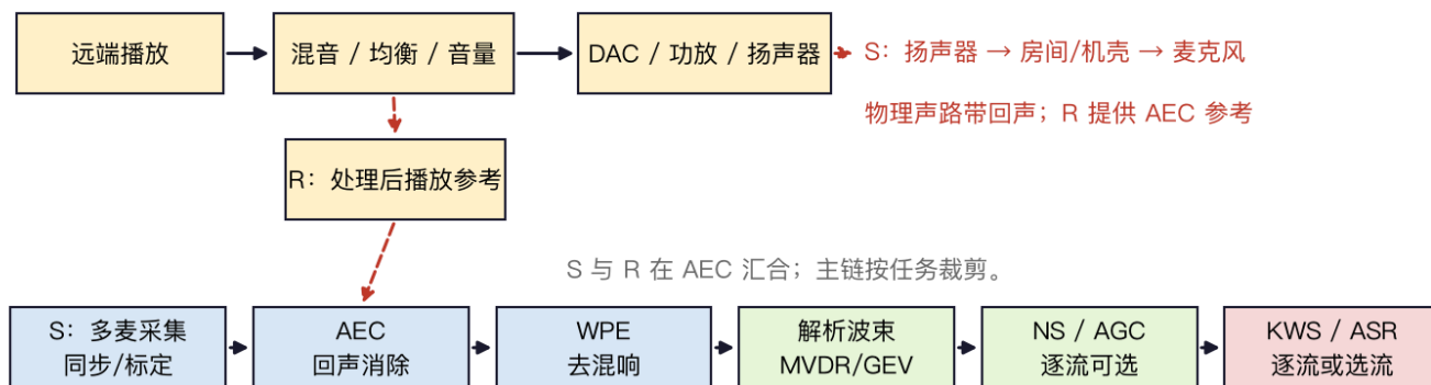
(a) 播放参考与音频主链
