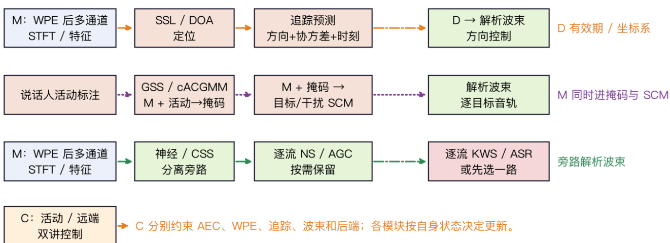
(b) 按任务选择的方向、GSS 与分离支路
