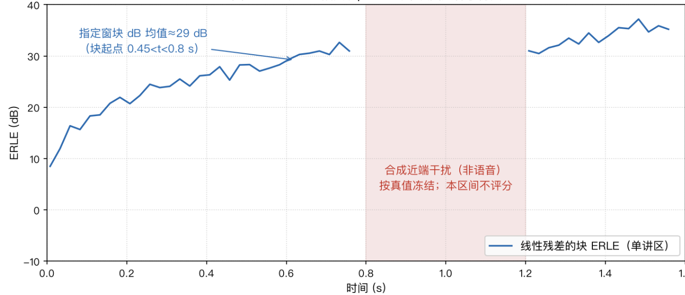
(b) 16 kHz、128 抽头、 \mu=0.5 的单次固定种子仿真
