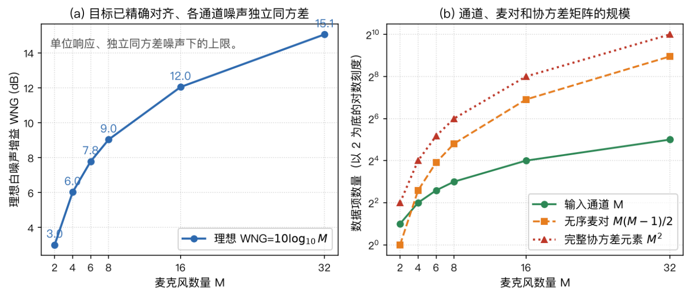
图9 麦克风数量增加时的理想增益与数据项数量 (公式计算，不给出产品选型排名)
