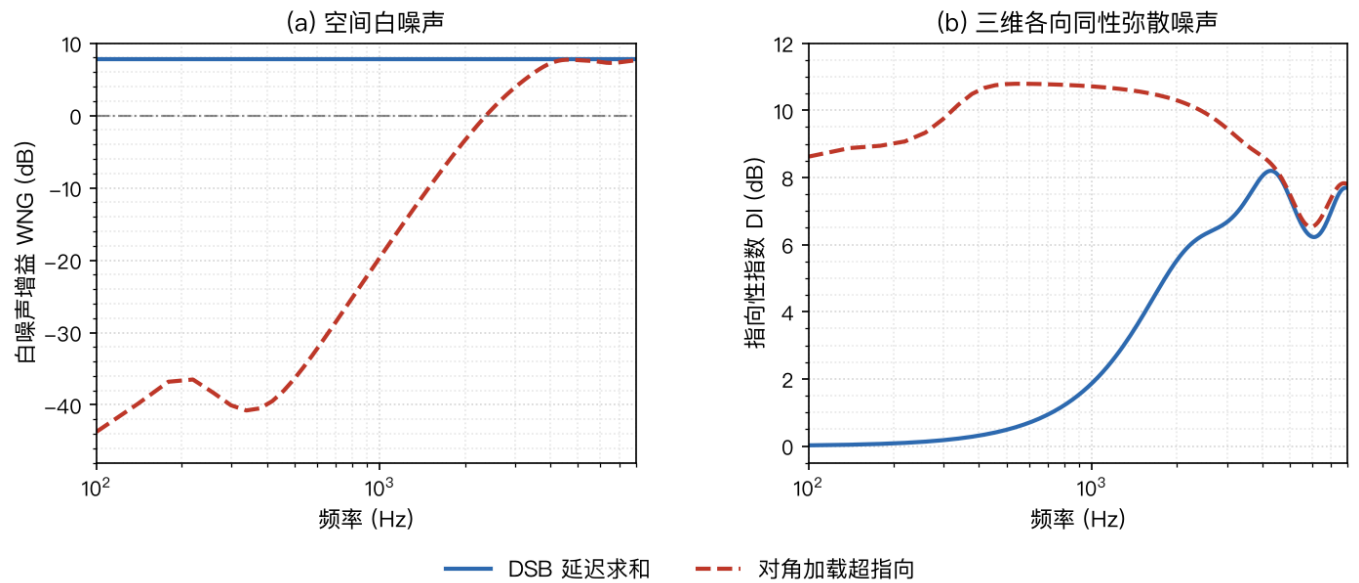
图15 6 麦圆阵的白噪声增益与指向性 半径与相邻弦长均为 4 cm；朝向 +x（正横角 90^\circ ）；声速 343 m/s 超指向采用相对对角加载 10^{-6} ；使用未加载的弥散协方差计算 DI
