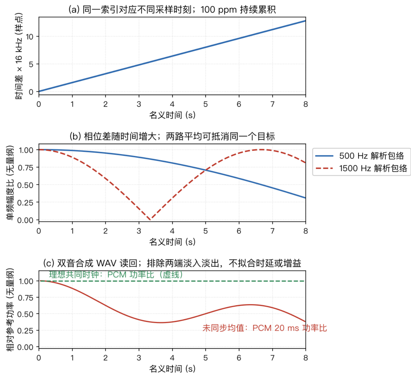
图 40: 16 kHz、100 ppm、8 s 数学合成例子；各文件采用同一导出增益。参考信号、双设备采样、未对齐均值与理想同步均值用于区分时钟误差和空间噪声。请结合 音频清单 读取参数。
