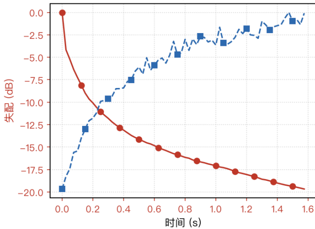
(b) 失配下降，ERLE 上升
