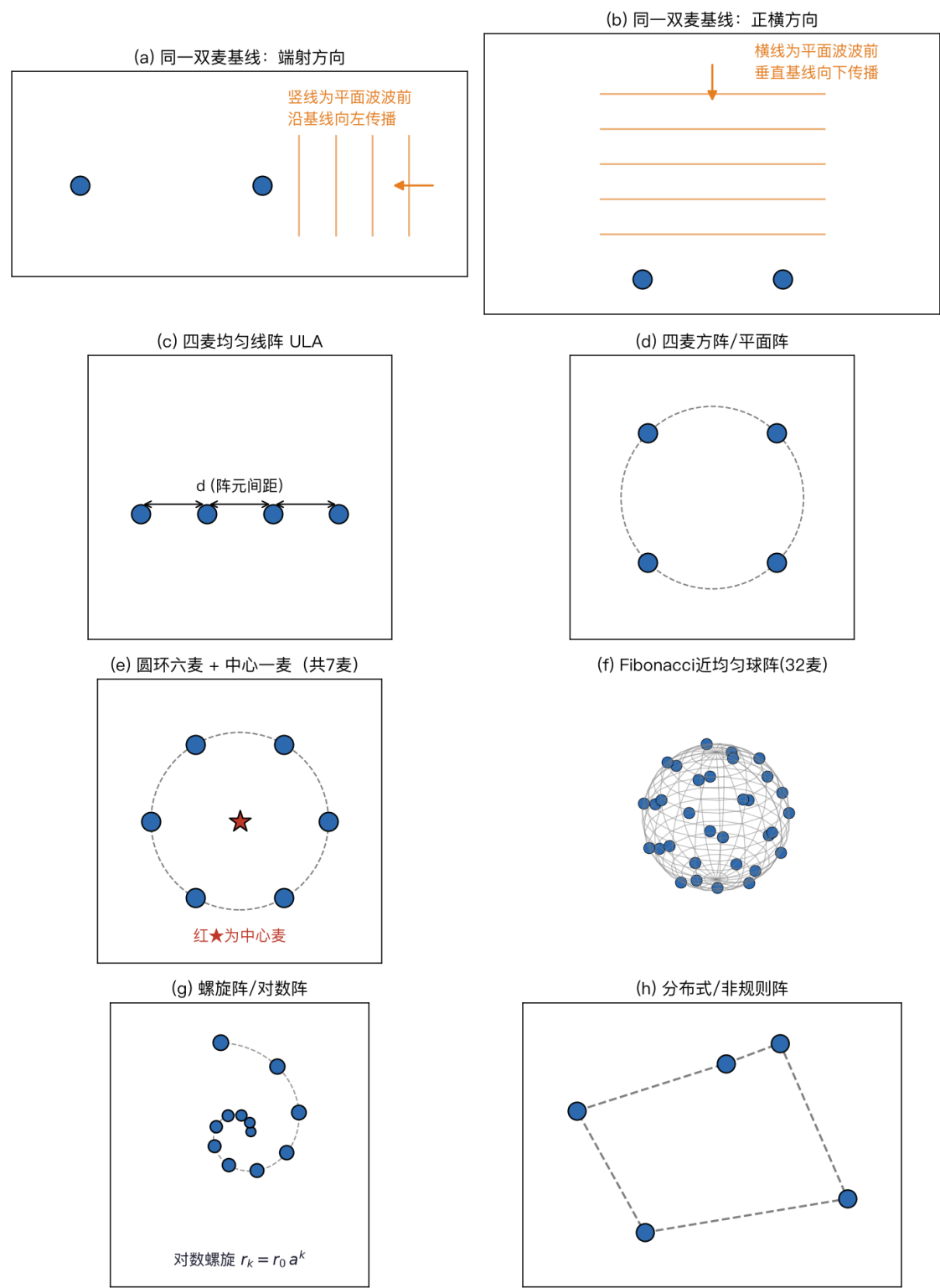
图8 常见麦克风阵列几何形态示意
