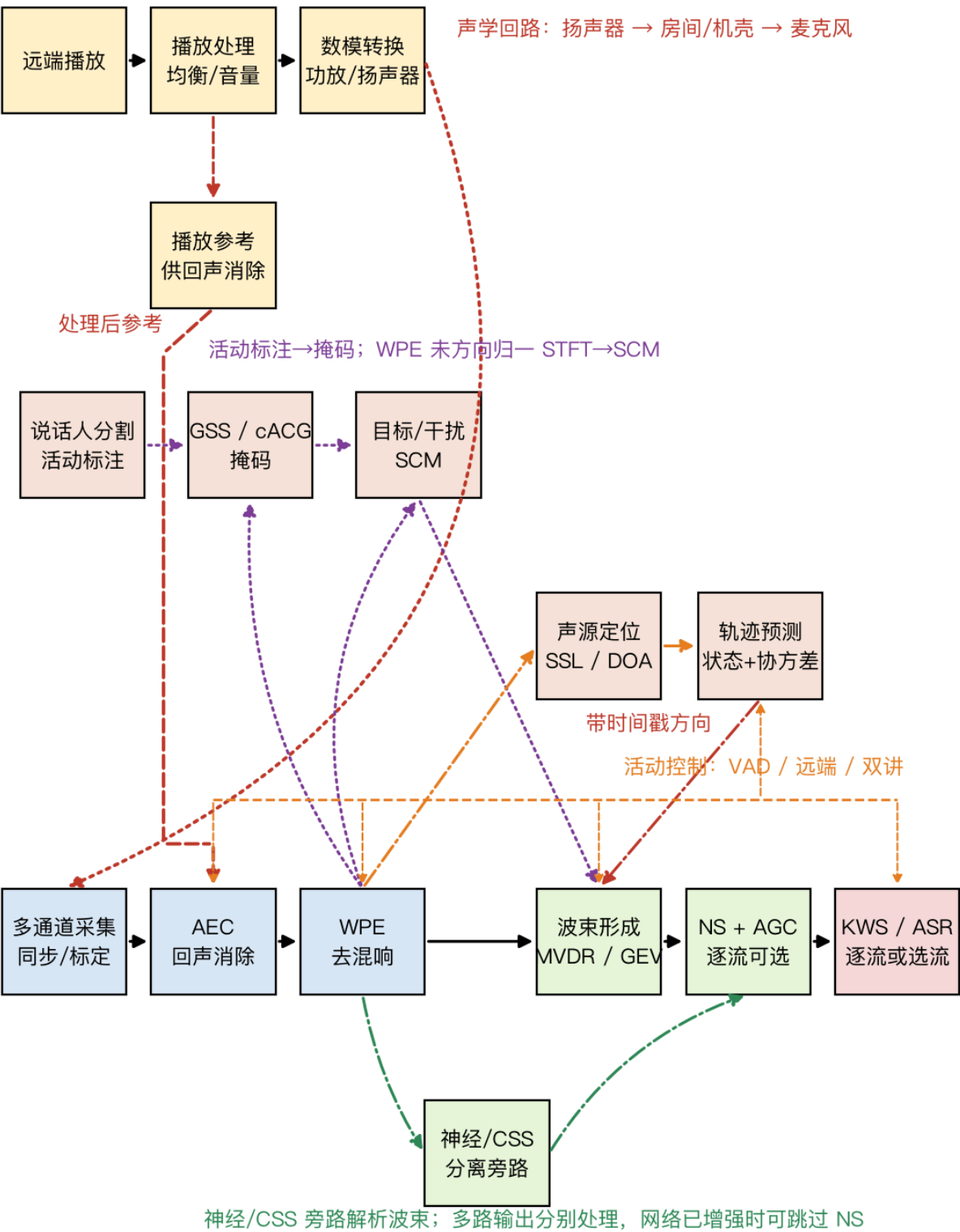
图 23 按较完整的语音交互系统绘制。远端音频先经过混音、均衡和音量控制；AEC 使用的播放参考取点位于这些处理之后、数模转换器（Digital-to-Analog Converter，DAC）和功率放大器之前。这样，参考信号包含实际播放时的混音与电平变化。
