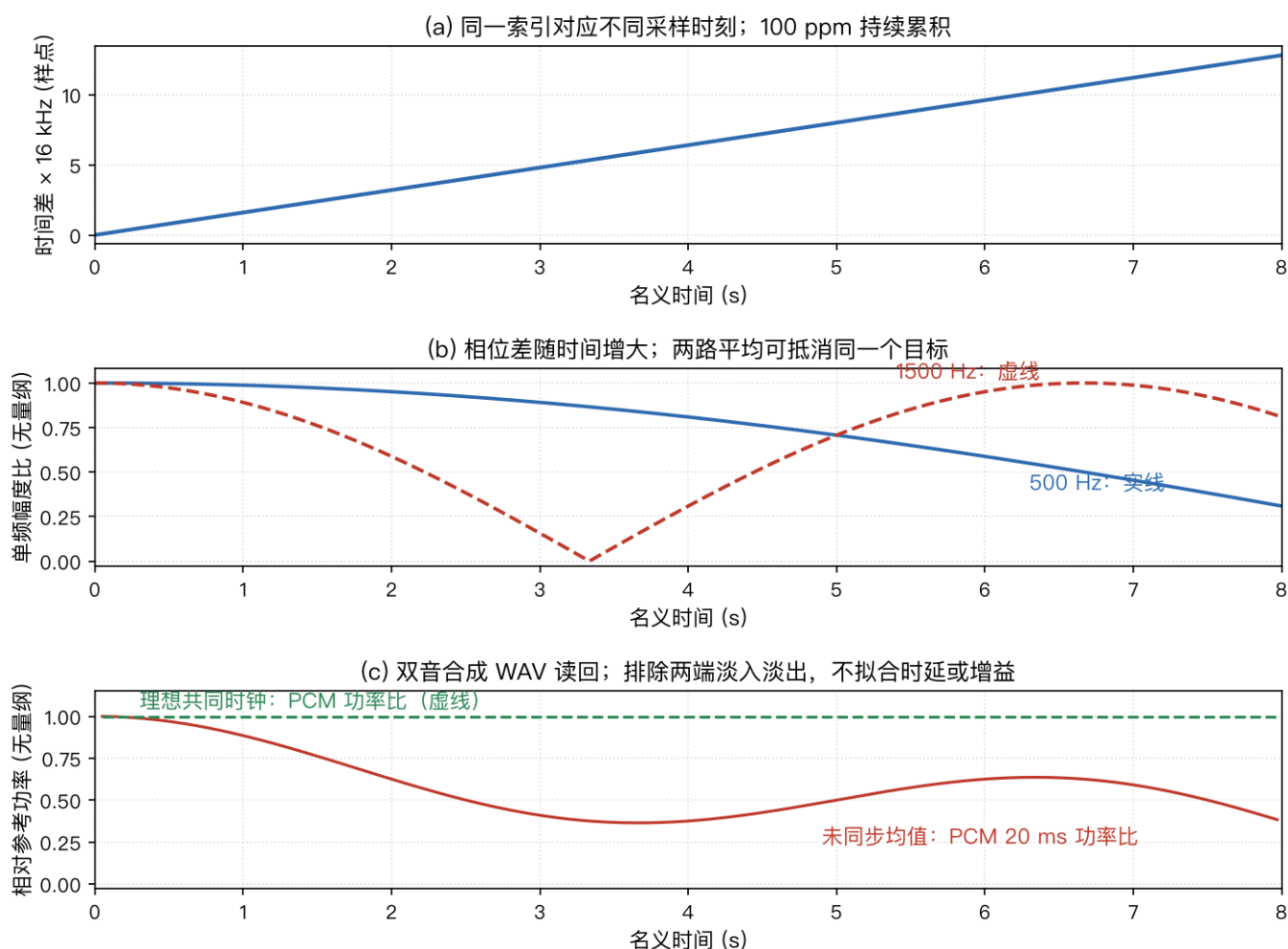
图 40：16 kHz、100 ppm、8 s 数学合成例子；各文件采用同一导出增益。参考信号、双设备采样、未对齐均值与理想同步均值用于区分时钟误差和空间噪声。请结合 音频清单 读取参数。
