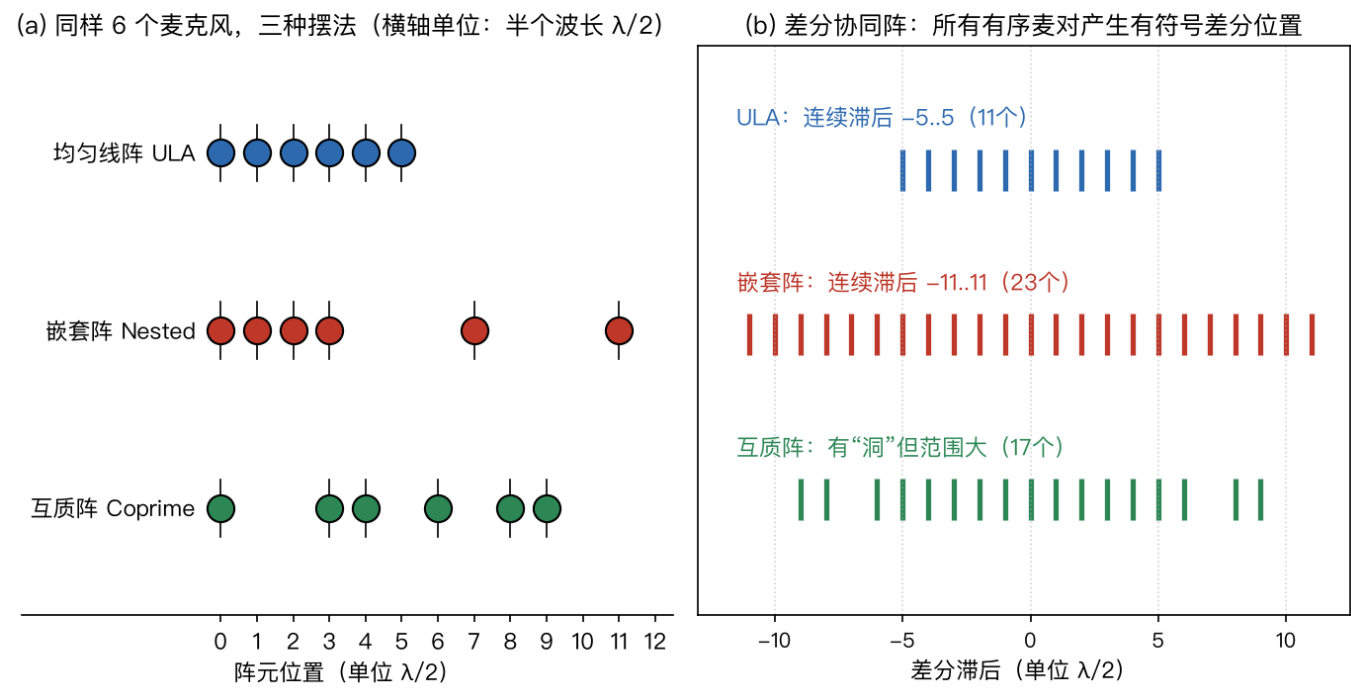
图10 稀疏阵列：6 个物理麦克风对应不同的有符号差分位置（模拟）
