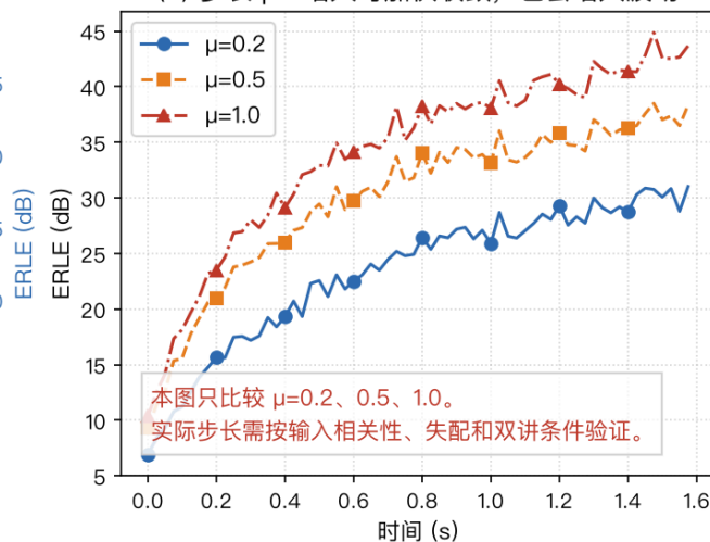
(c) 步长 \mu : 增大可加快收敛, 也会增大波动
