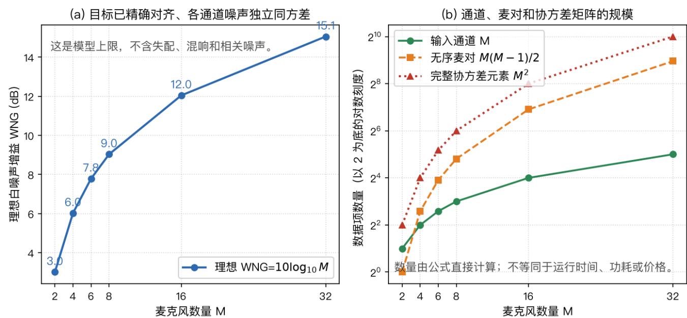
图 9 (a) 在目标精确对齐、各通道噪声独立同方差的条件下，按 10 \log_{10} M 画出理想 DSB 白噪声增益。(b) 分别按 M 、 M(M-1)/2 和 M^2 计算输入通道、无序麦对与完整协方差矩
