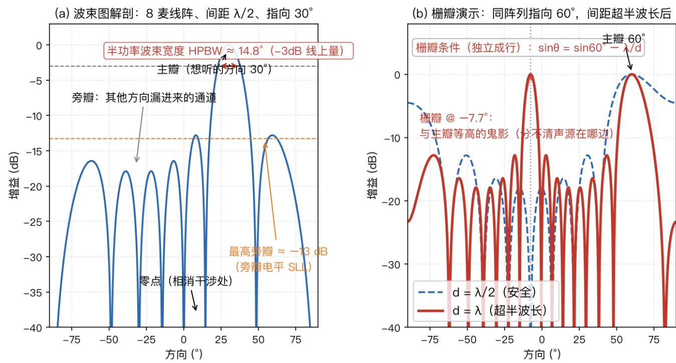
图7 波束图怎么读：主瓣 / HPBW / 旁瓣 / 零点 / 栅瓣（模拟）
