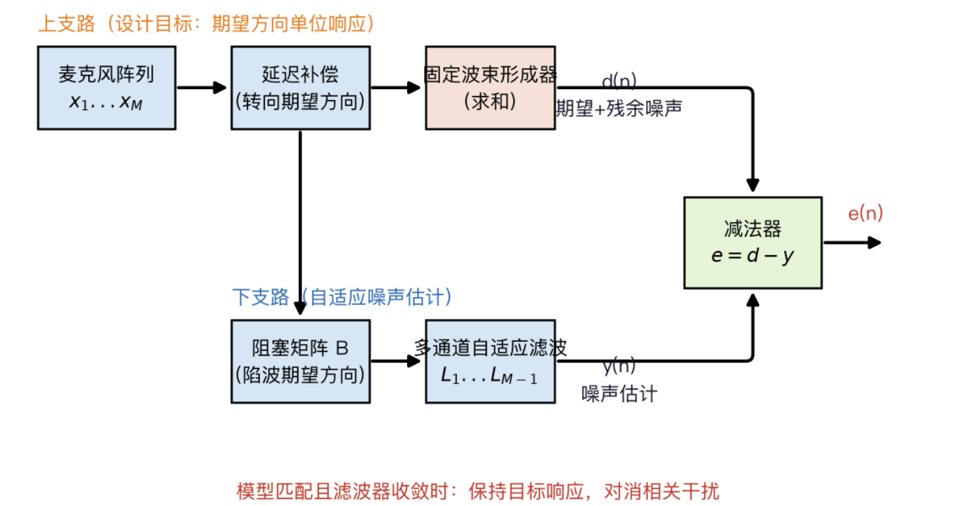
图17 GSC（广义旁瓣对消器）结构框图
