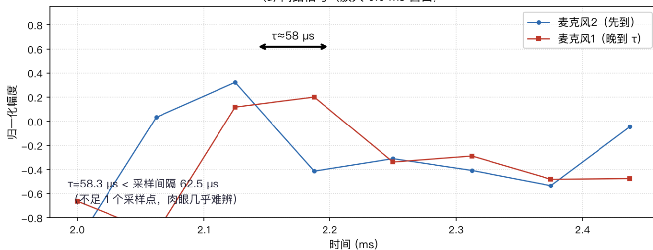
(a) 两路信号（放大 0.5 ms 窗口）
