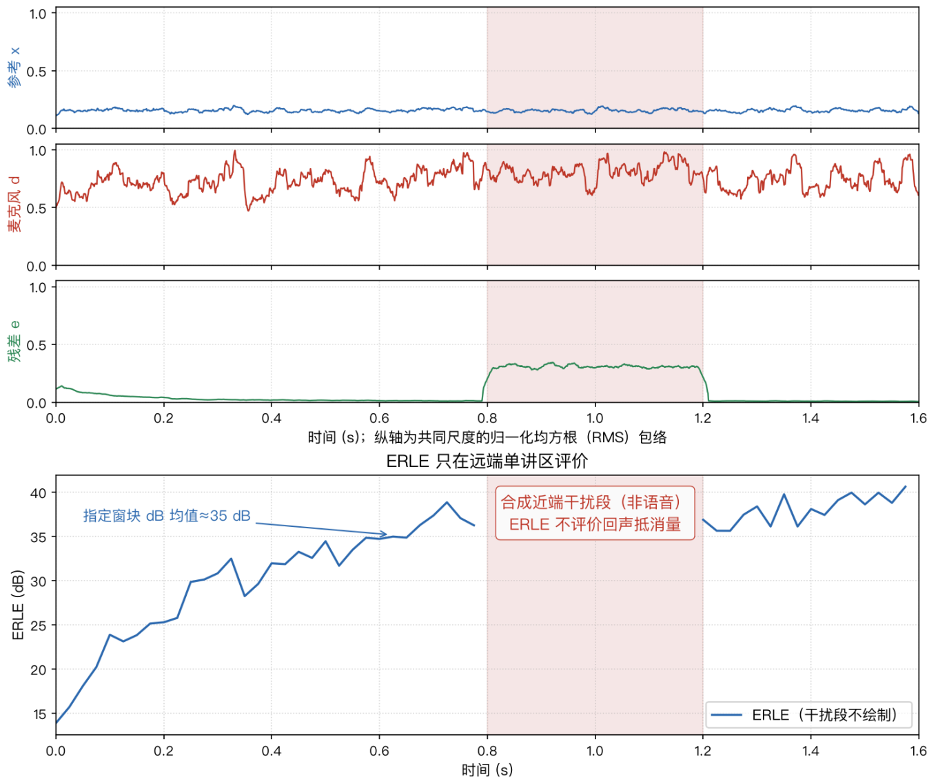
图29 NLMS 收敛与合成近端干扰时的冻结
